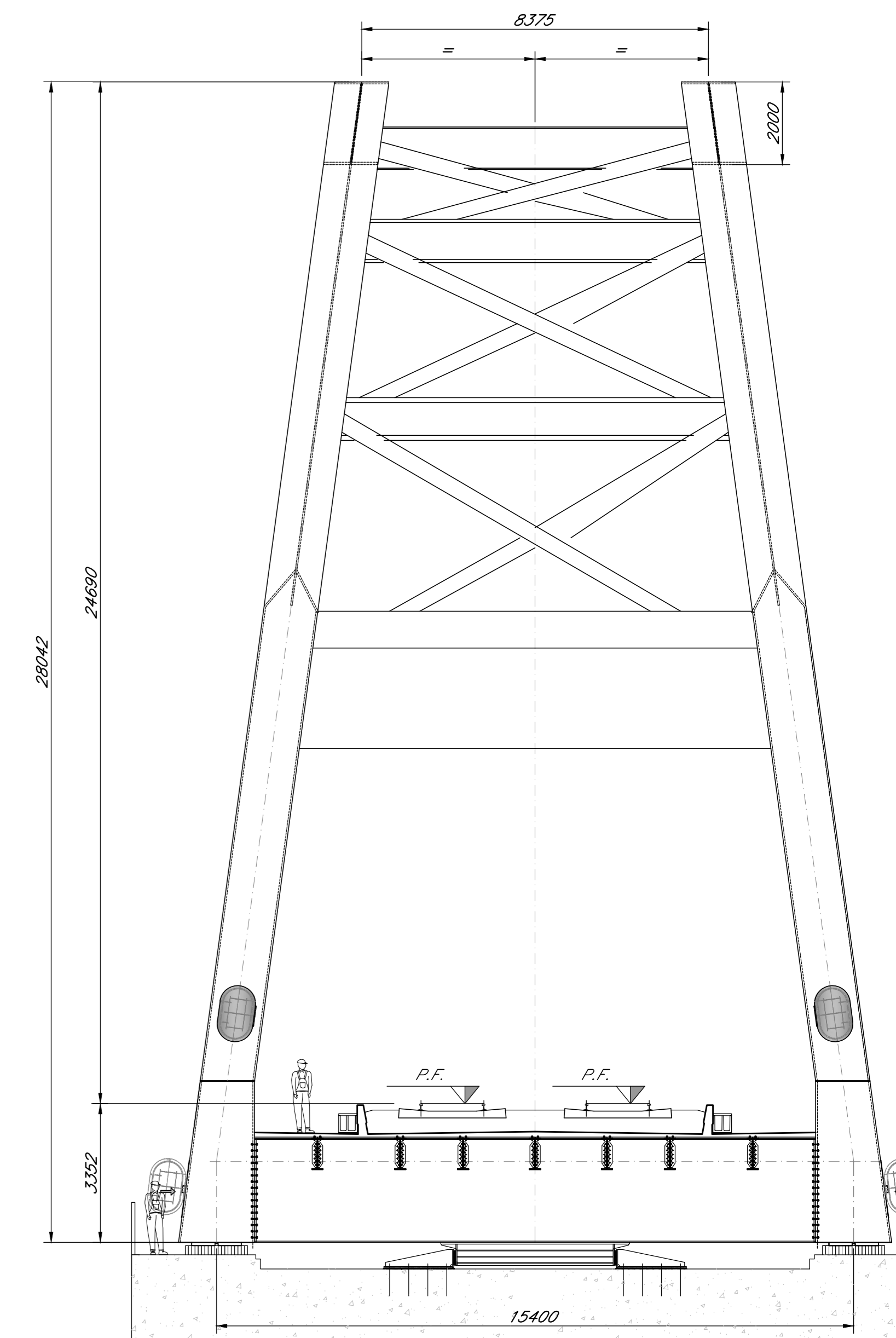
SEZIONE TRASVERSALE Scala 1:100
