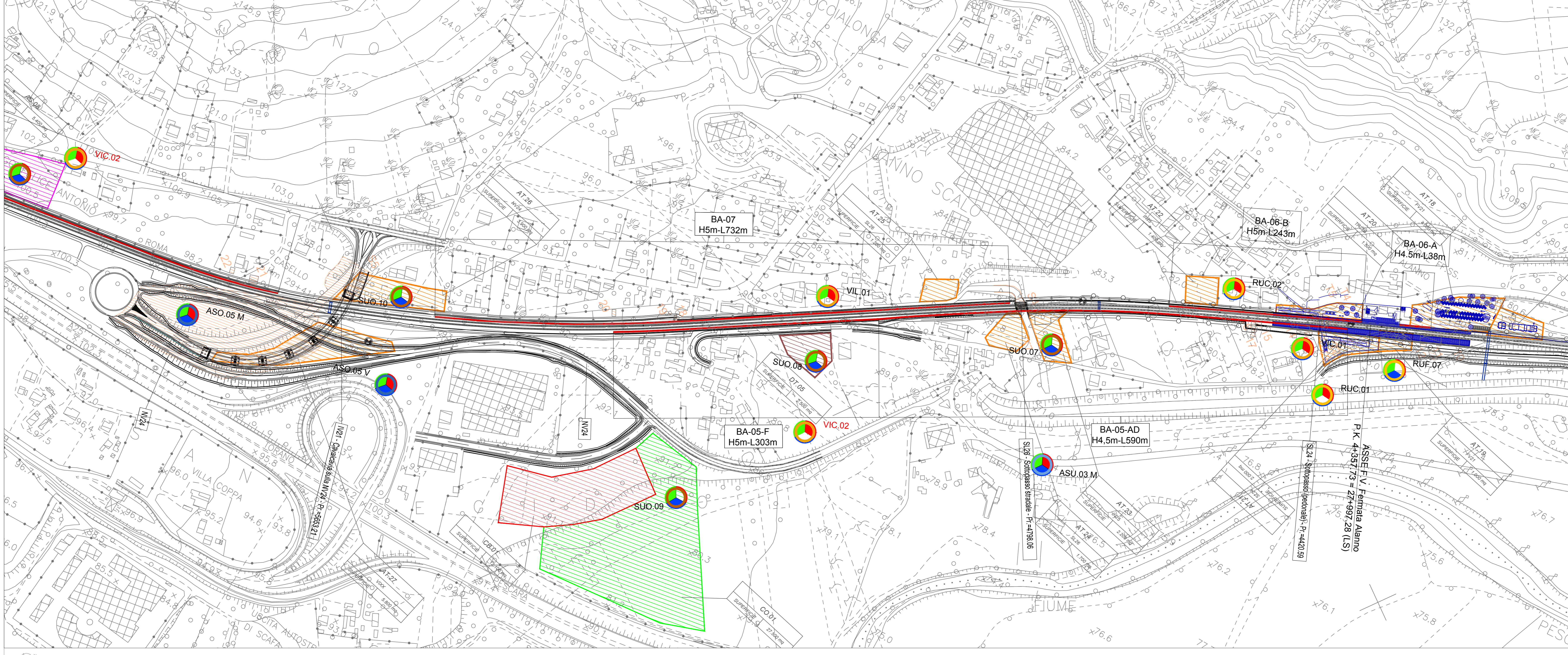
TRATTO D - PLANIMETRIA DI LOCALIZZAZIONE DEI PUNTI DI MONITORAGGIO
