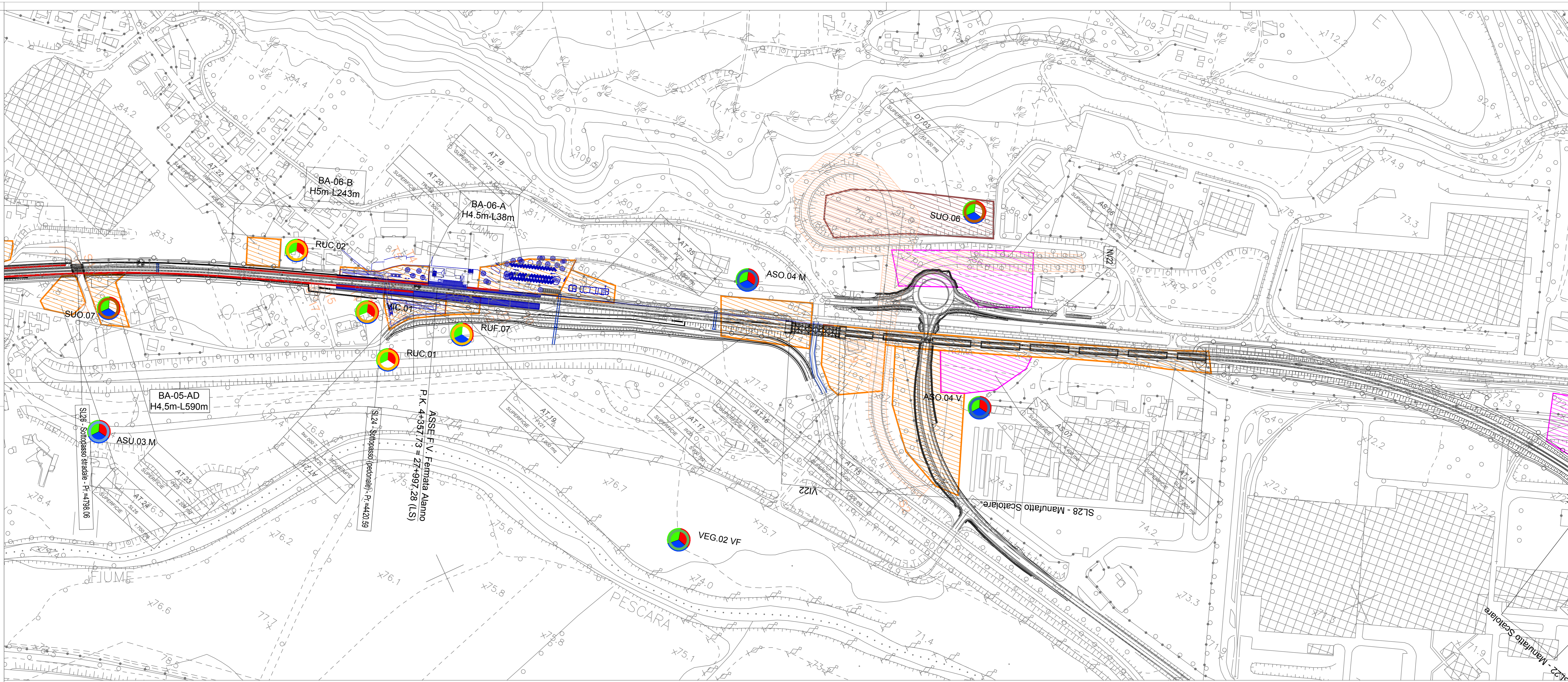
TRATTO C - PLANIMETRIA DI LOCALIZZAZIONE DEI PUNTI DI MONITORAGGIO
