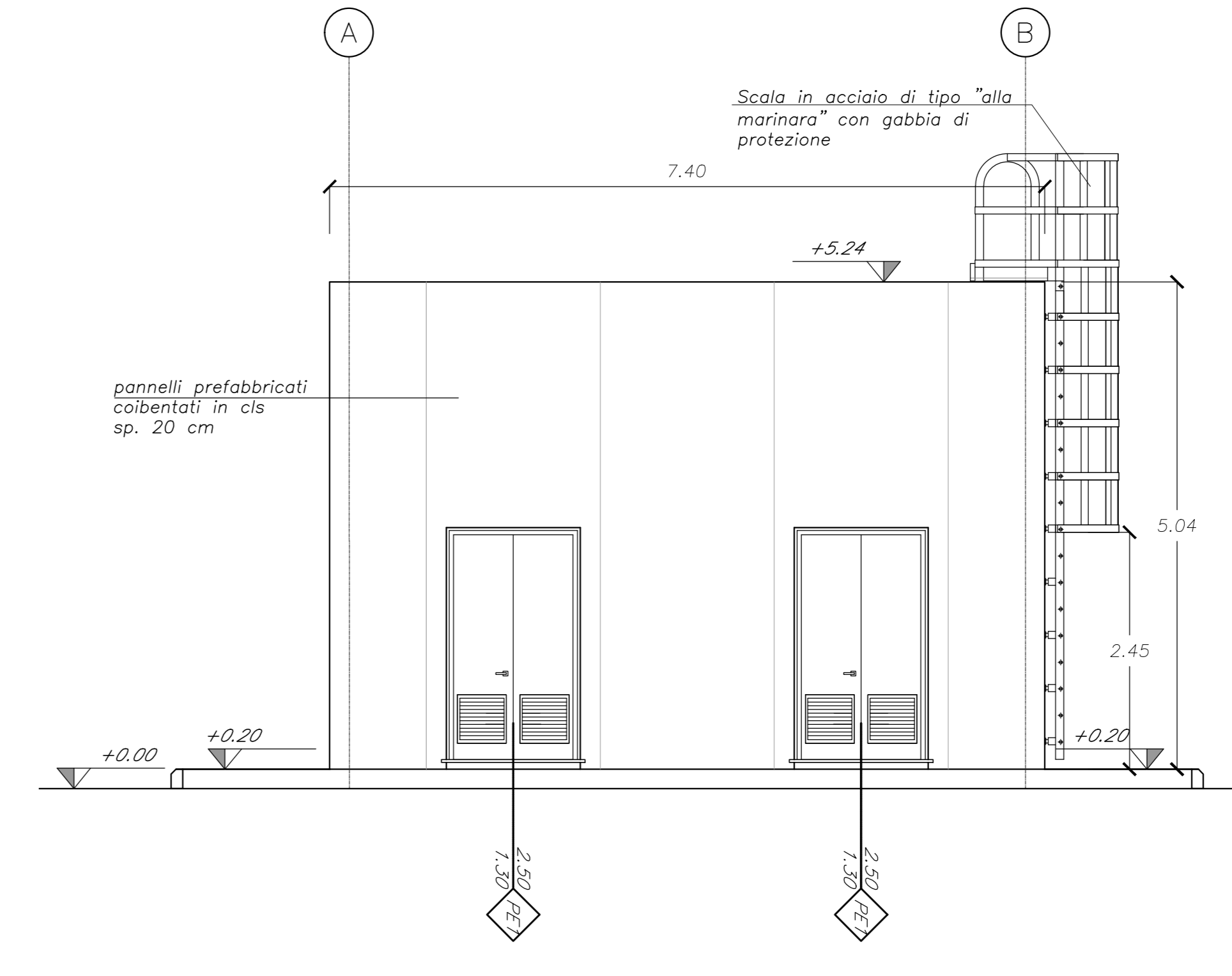
Prospetto 4 Scala 1:50
