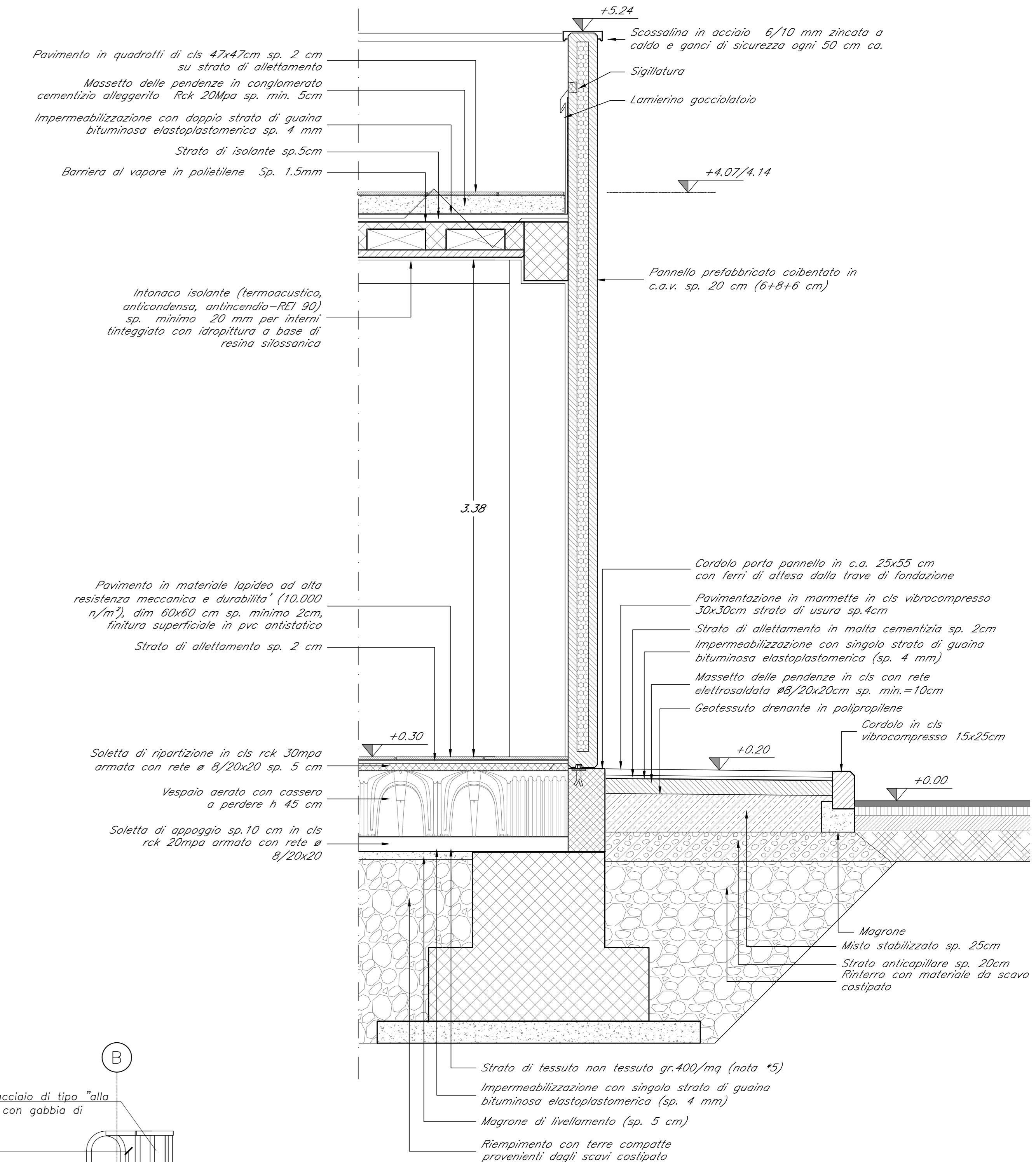
Sezione tipo Scala 1:20
