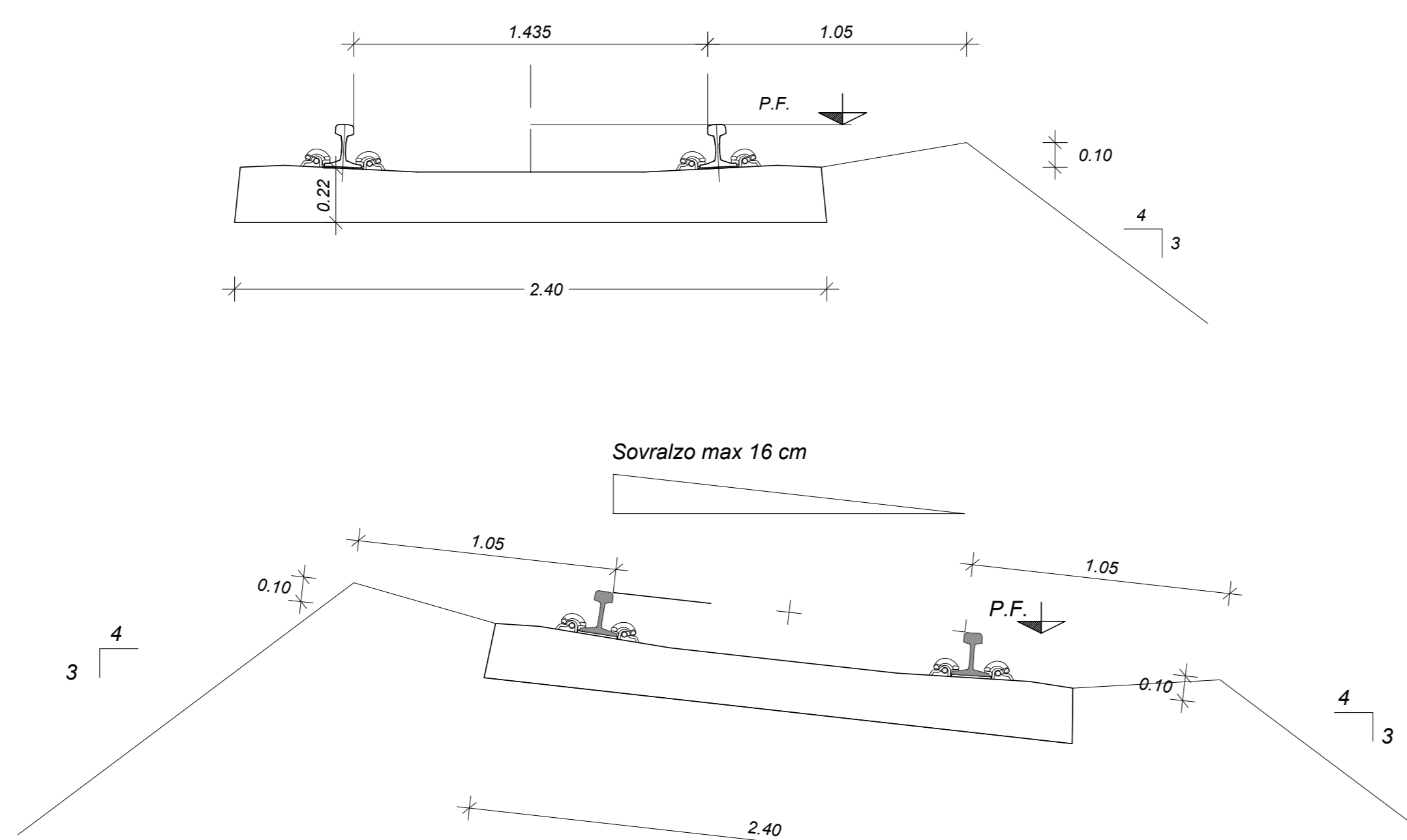
Dettaglio "1" - Andamento traversa in rettilineo ed in curva
