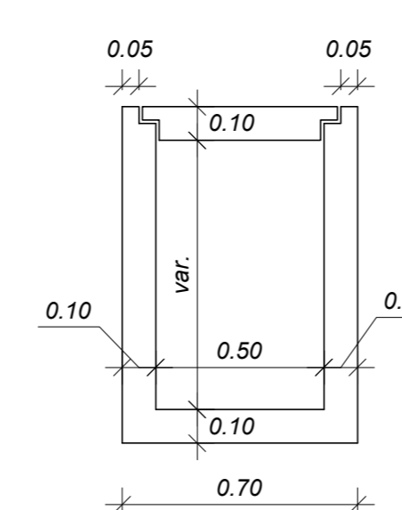
Dettaglio "2" - Canaletta idraulica
