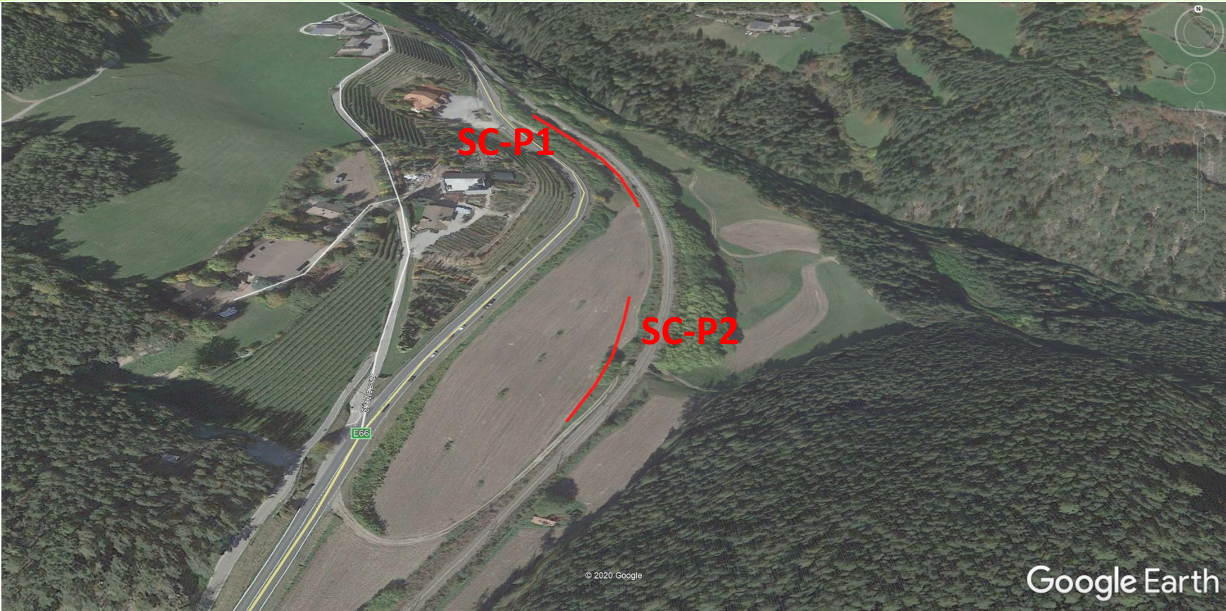
Vista tridimensionale da Sud dei profili sismici a rifrazione SC-P1 e SC-P2
