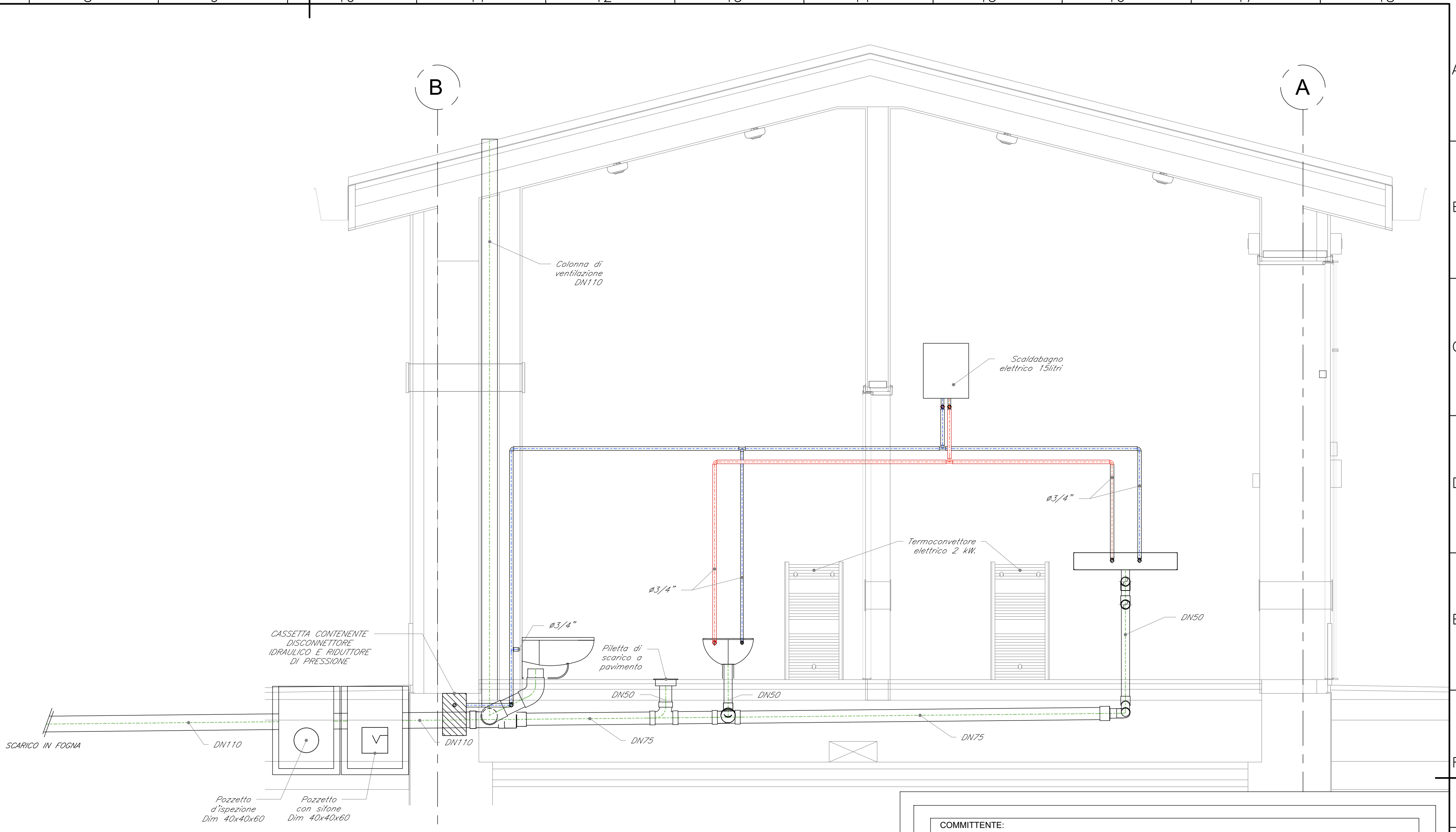
SEZIONE A-A
