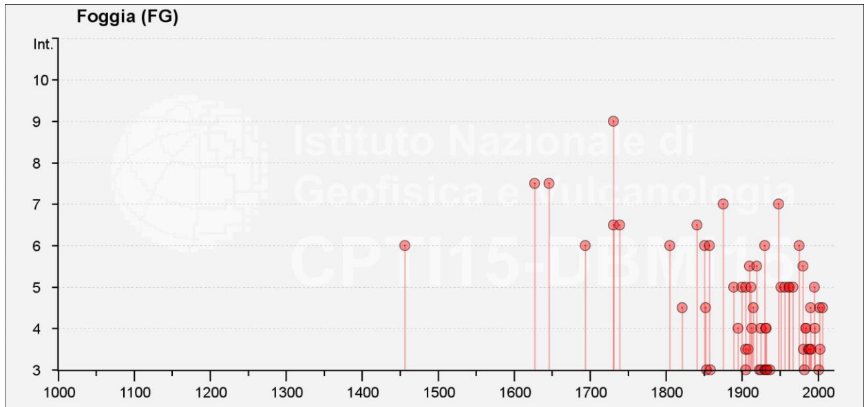
Figura 20 – Storia sismica del Comune di Foggia [41.462, 15.545] – https://emidius.mi.ingv.it/CPTI15-DBMI15_v1.5/query_place/
