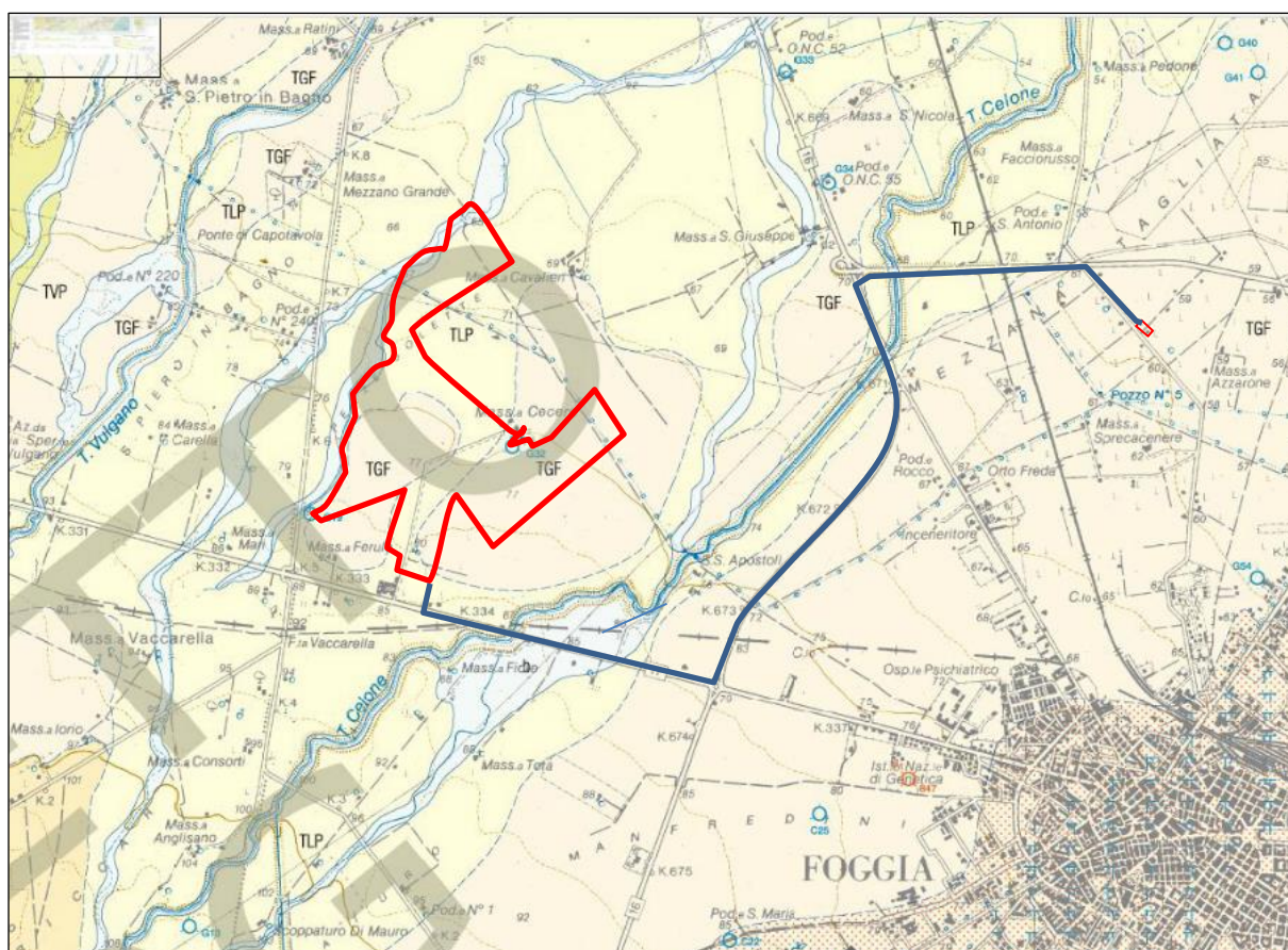
Figura 9 – Estratto della Carta Geologica Foglio 408 Foggia - Nel riquadro l'area di insediamento dell'impianto fotovoltaico e della Stazione Elettrica
