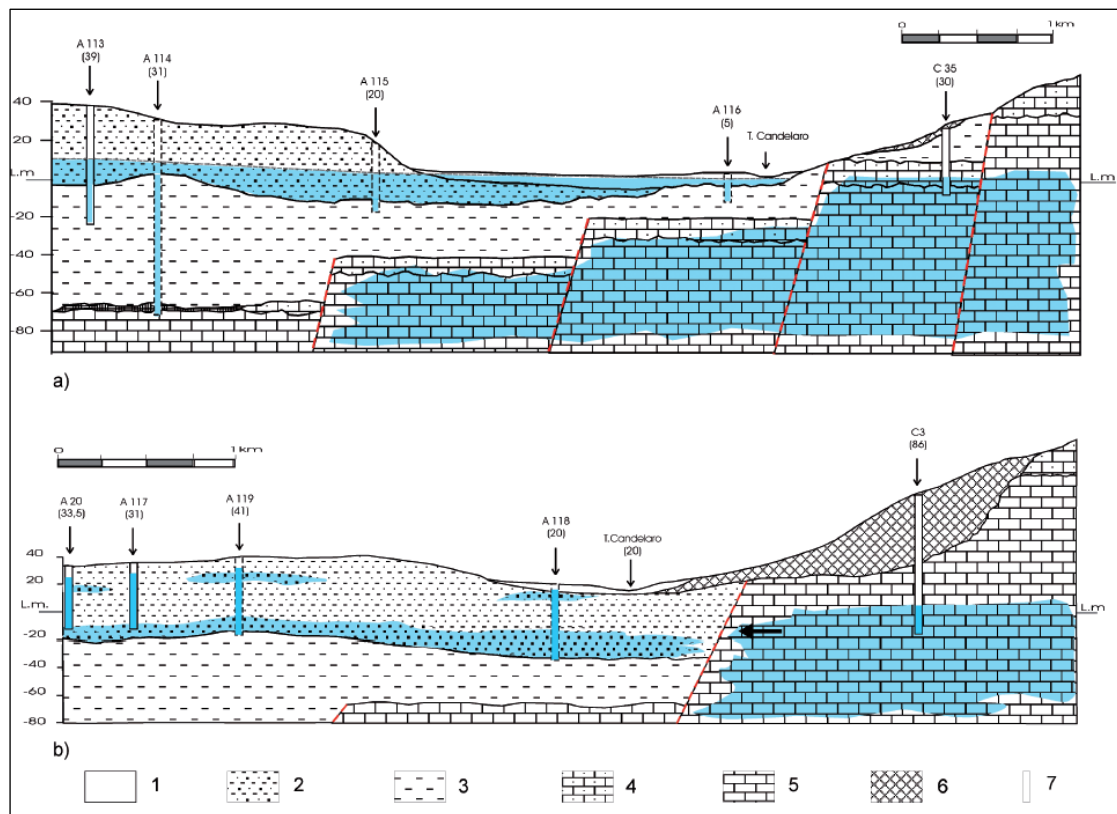
Figura 15 – Sezioni idrogeologiche. Legenda 1) Depositi d'alveo (Olocene); 2) depositi della pianura alluvionale (Olocene – Pleistocene sup.); 3) argille grigio- azzurrognole con intercalazioni sabbiose (Pleistocene inf. – Pliocene sup.) 4) Calcarenite (Pliocene sup. – Miocene); calcari della piattaforma carbonatica apula (Cretaceo); 6) Conoidi detritiche (Olocene – Pleistocene sup.) 7) Pozzo (in tratteggio, se proiettato).
