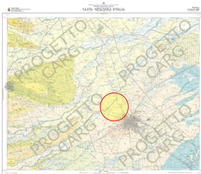
Figura 4 – Carta Geologica d'Italia - Foglio 408 Foggia.
