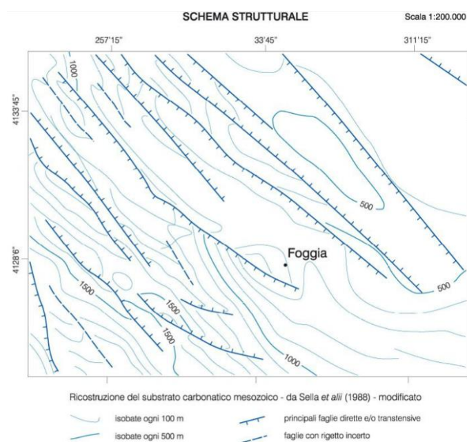
Figura 10 – Schema strutturale del foglio 408 – Foggia.
