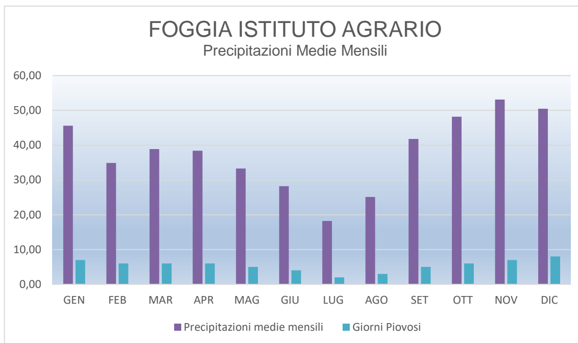
Figura 13 – Precipitazioni medie mensili e numero dei giorni piovosi nella stazione pluviometrica di Foggia Istituto Agrario 1946 - 2013.
