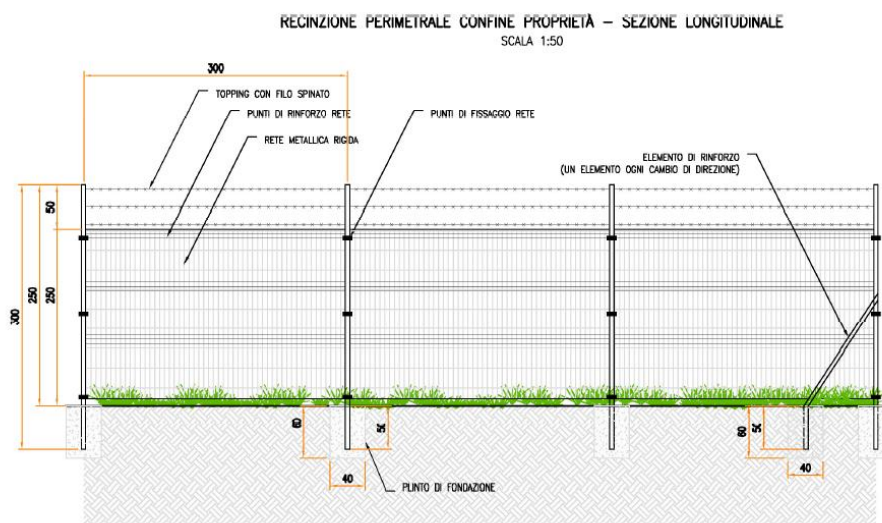
Figura 2.8: Particolare recinzione
