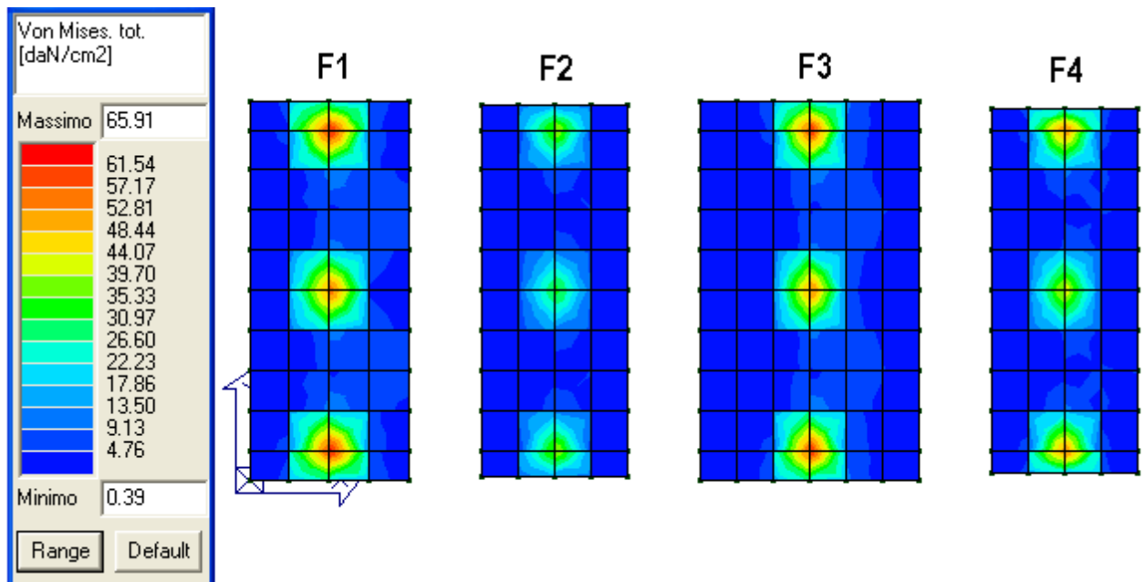
Mappa cromatica delle tensioni totali (membrana + flessione) ottenute mediante la formulazione di Von Mises - Comb. SLE rara
