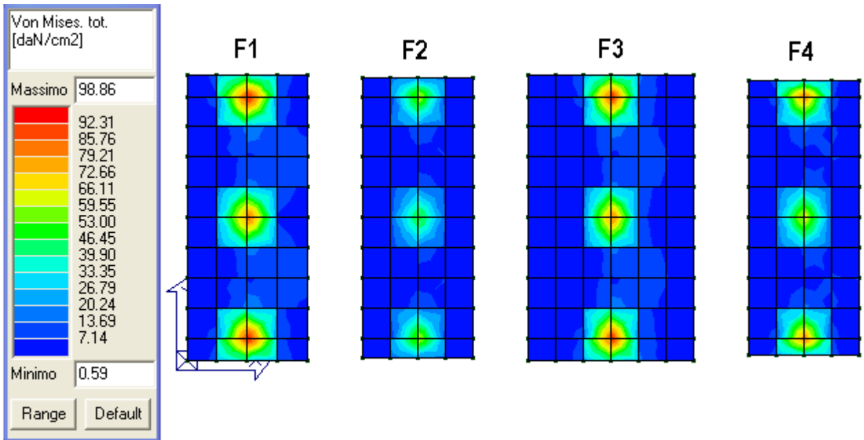
Mappa cromatica delle tensioni totali (membrana + flessione) ottenute mediante la formulazione di Von Mises - Comb. SLU
