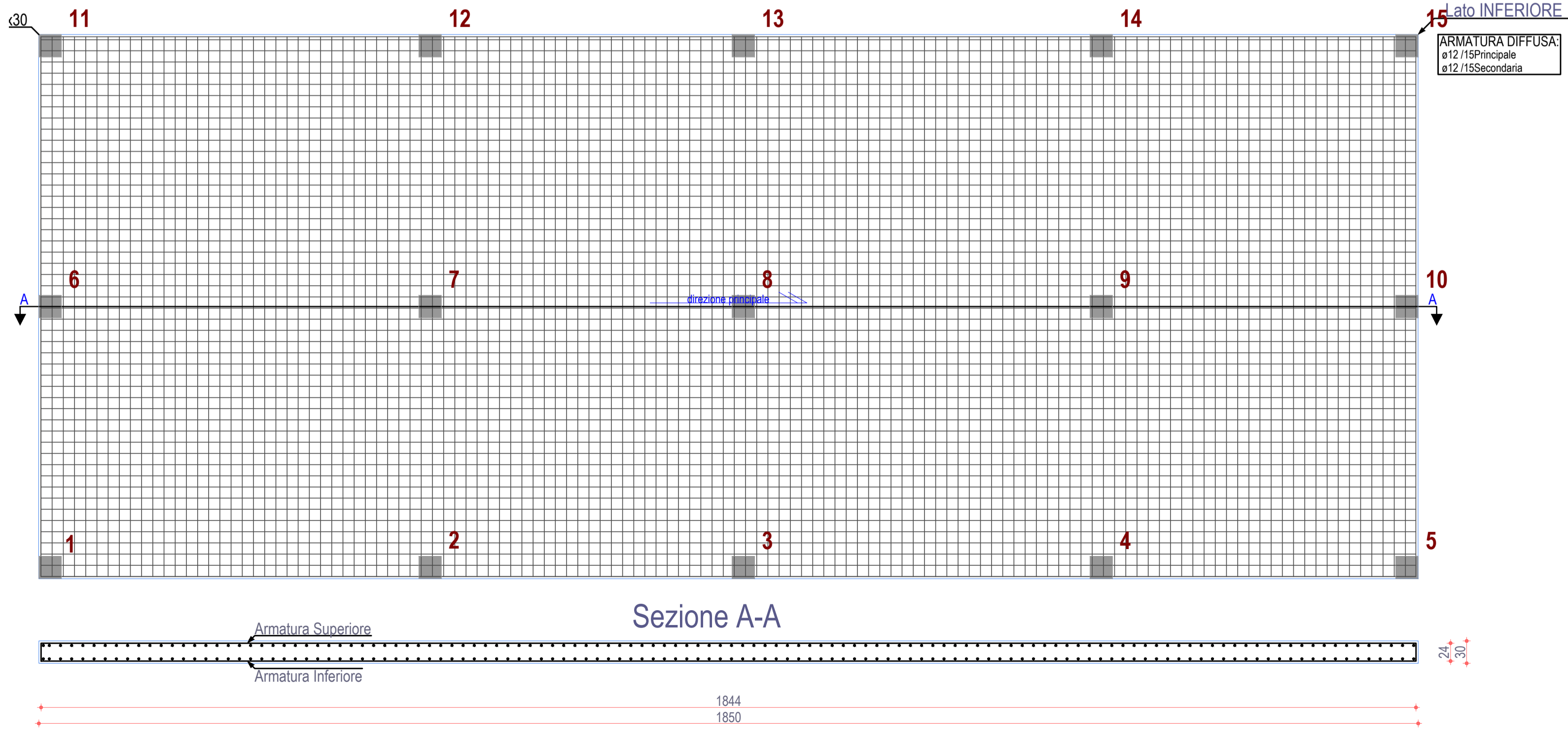
PLATEA SCALA 1:50
