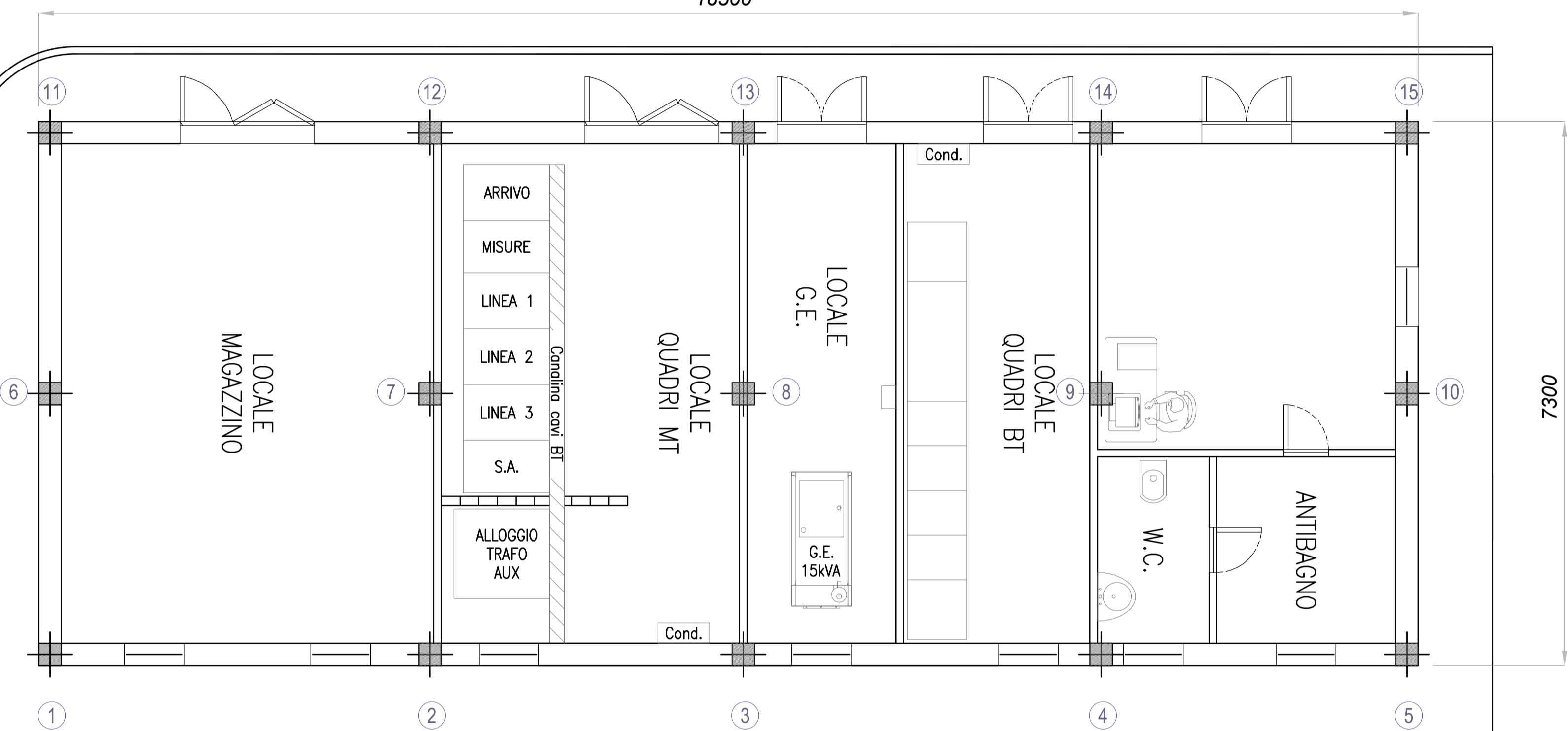
PIANTA SCALA 1:50
