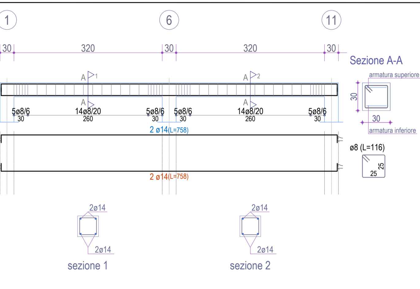
TRAVE 1-11,2-12,3-13,4-14,5-15 SCALA 1:50
