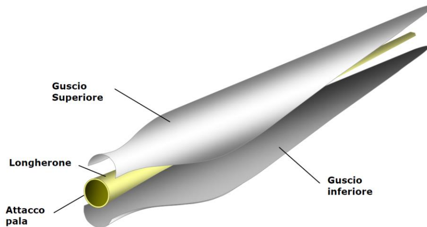
Figura 1 Composizione di una pala
