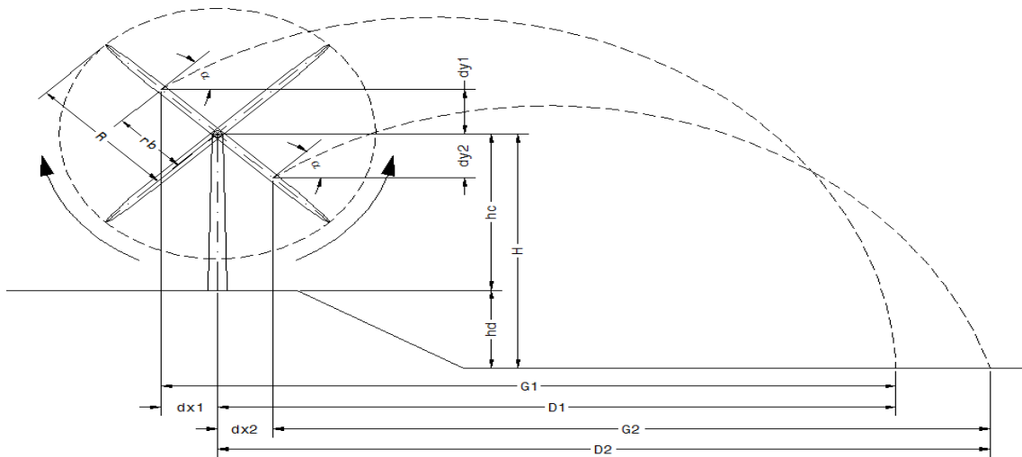
Figura 3 Schema grafico di gittata
