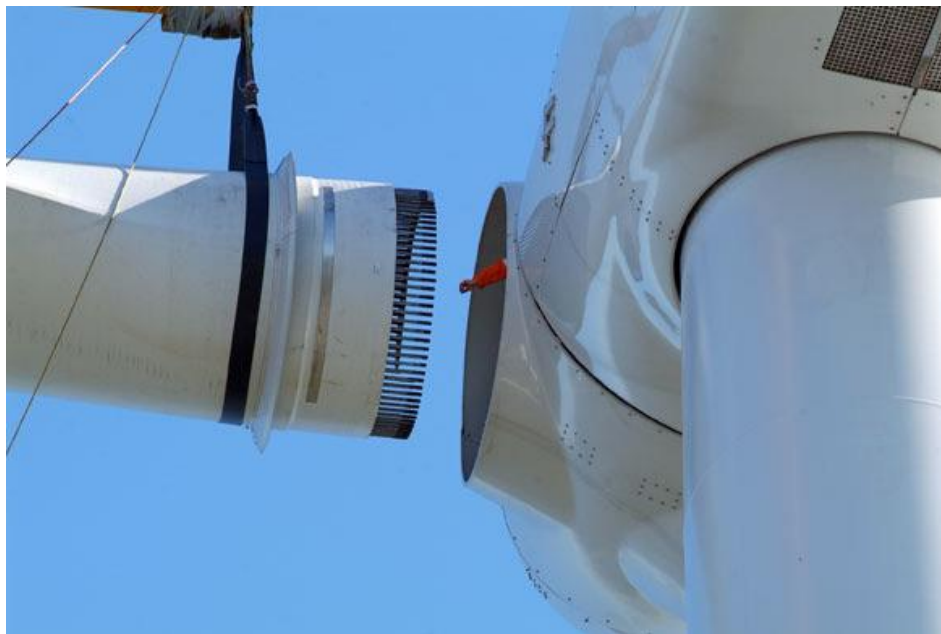
Figura 2 Collegamento pala-mozzo
