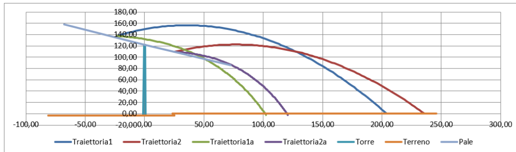
Figura 9 Calcolo della gittata mediante interpolazione dei diversi valori assunti dall'angolo di lancio \alpha in REAL CASE considerando un dislivello in posizione sottomessa della turbina rispetto al ricevitore e la presenza di attrito viscoso dovuto all'aria
