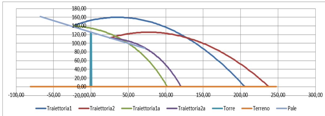
Figura 4 Calcolo della gittata mediante interpolazione dei valori assunti dall'angolo di lancio \alpha in WORST CASE
