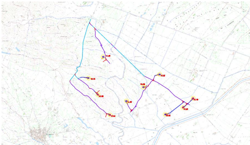
Figura 5 Inquadramento degli aerogeneratori proposti su CTR
