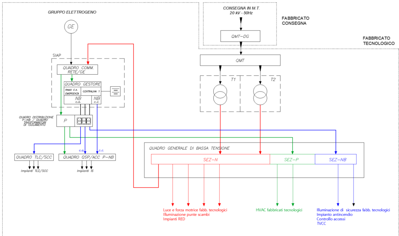
Figura 2 - Schema di alimentazione impianto elettrico lungo linea con consegna in media tensione PM Interporto D'Abruzzo
