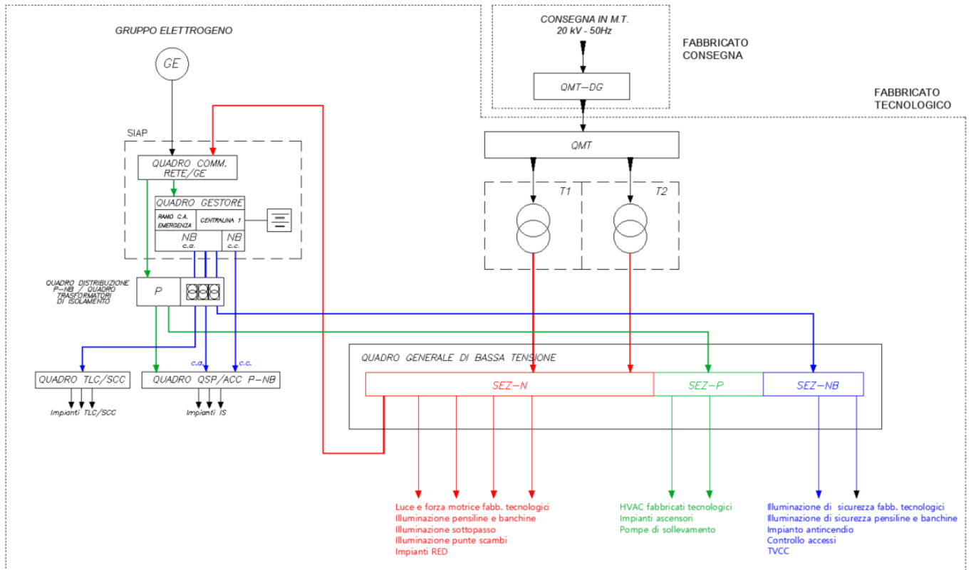
Figura 4 - Schema di alimentazione impianto elettrico di stazione con consegna in media tensione - Stazione di Manoppello
