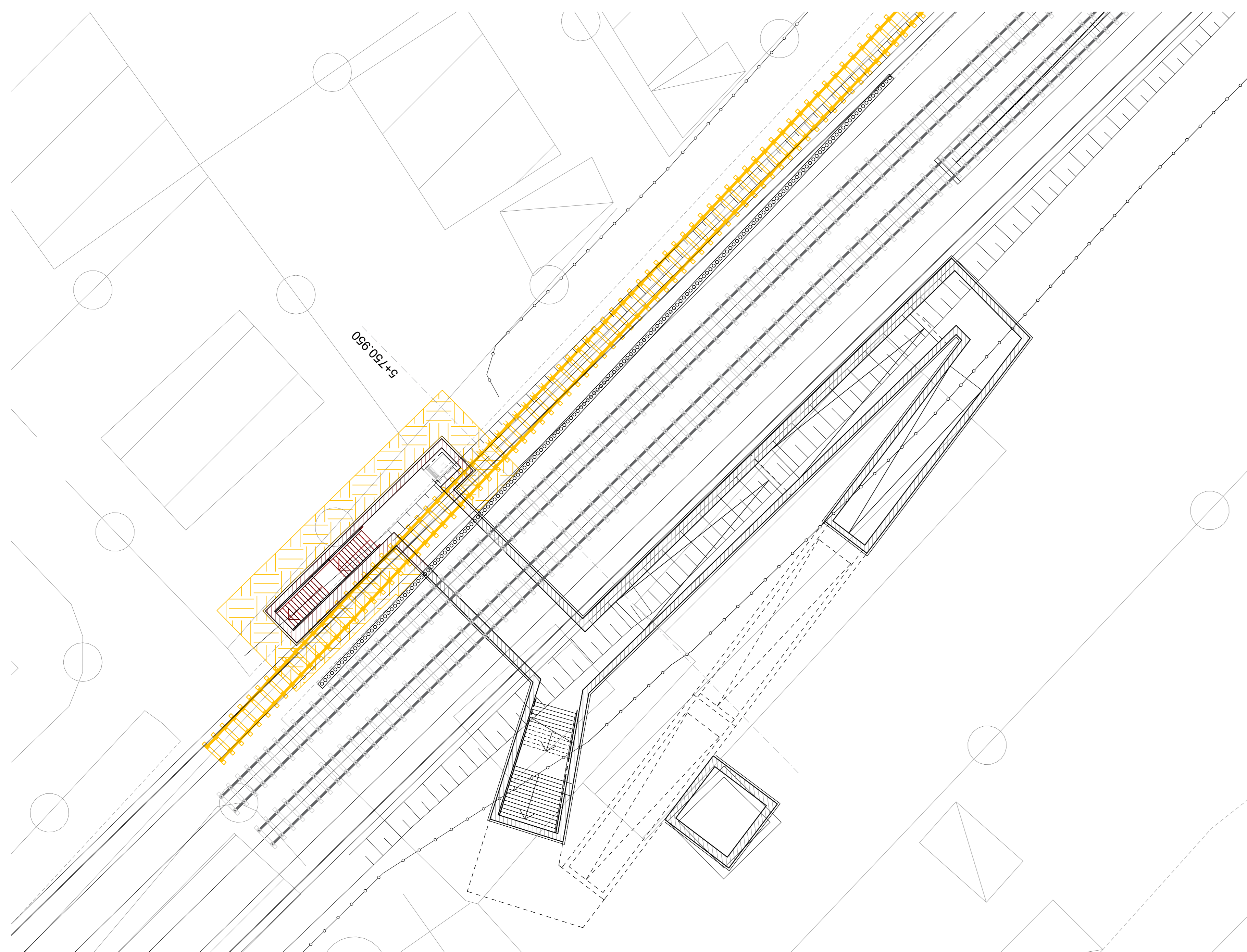
Fase 2 - Apertura nuova linea - Demolizione dei binari esistenti - Scavo e realizzazione delle opere
