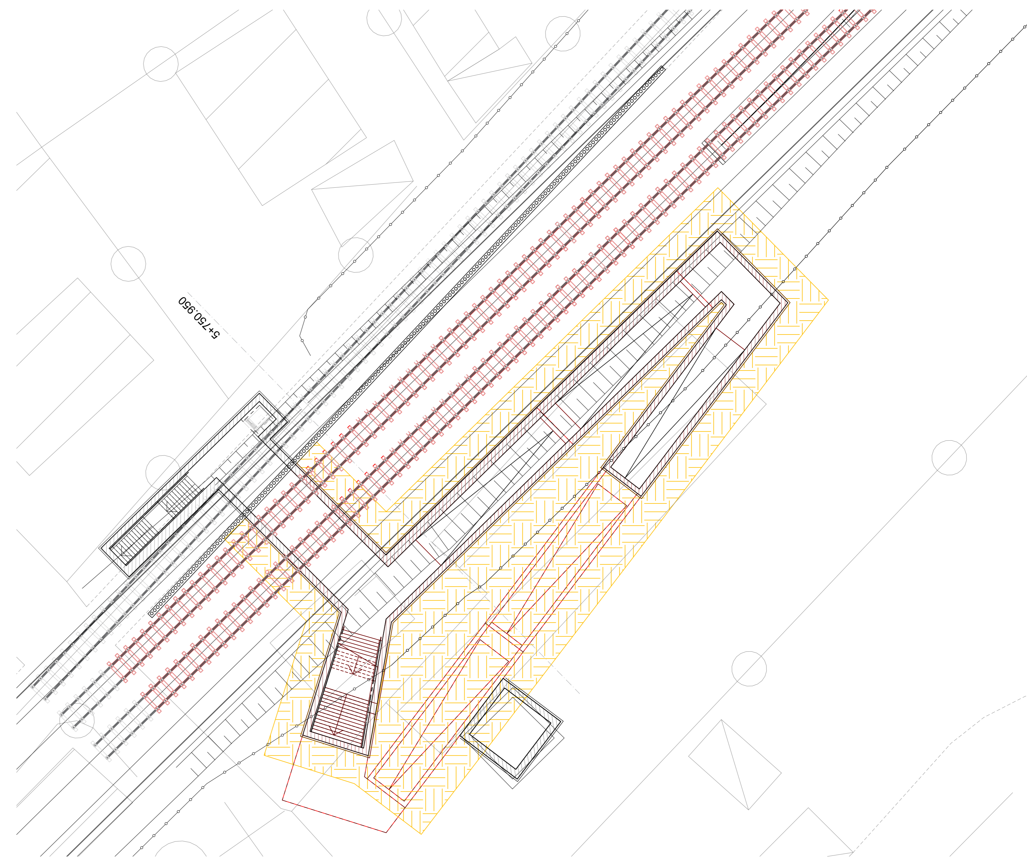
Fase 1 - Scavo e realizzazione delle opere a sud della tratta esistente - Realizzazione binari di progetto
