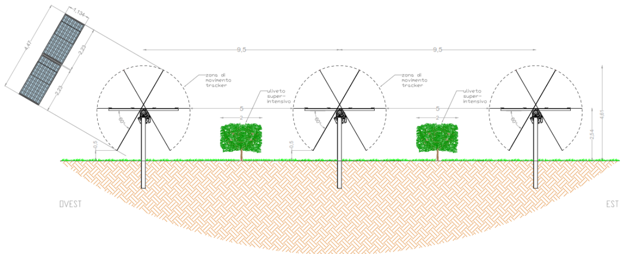
Fig. n°1 Sistema Agro-fotovoltaico
