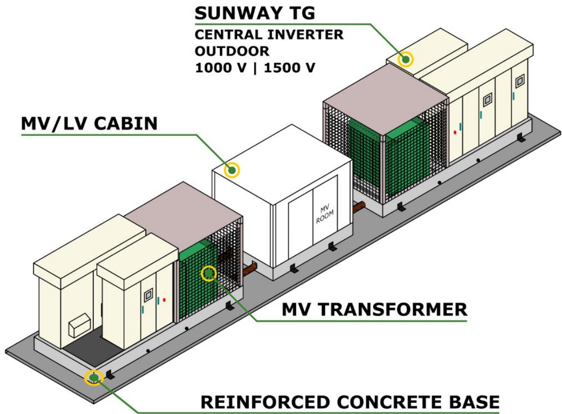
Fig. n°17 Power Skid
