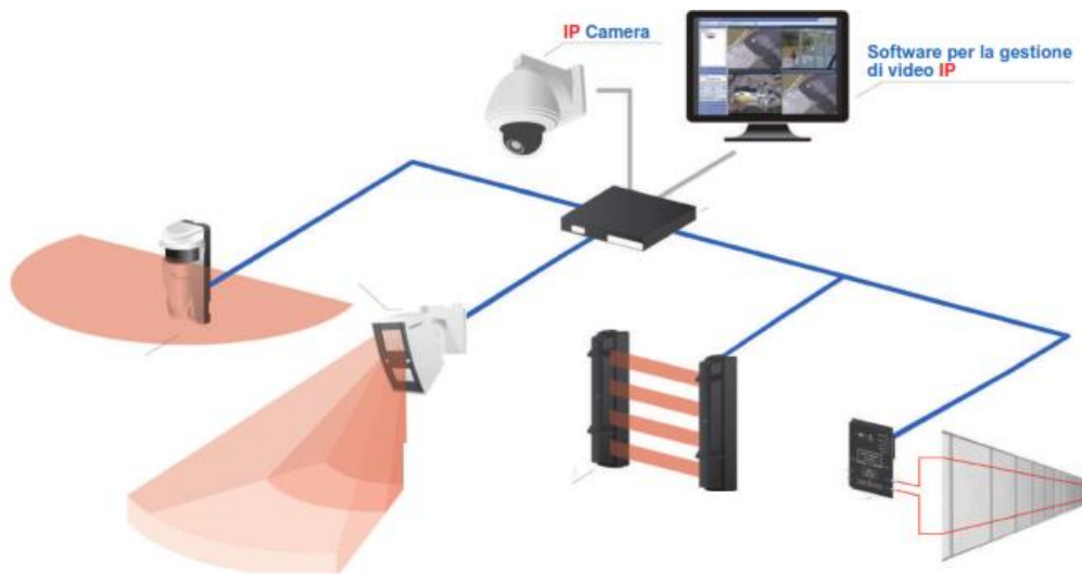
Fig. 27 Sistema di videosorveglianza e antintrusione
