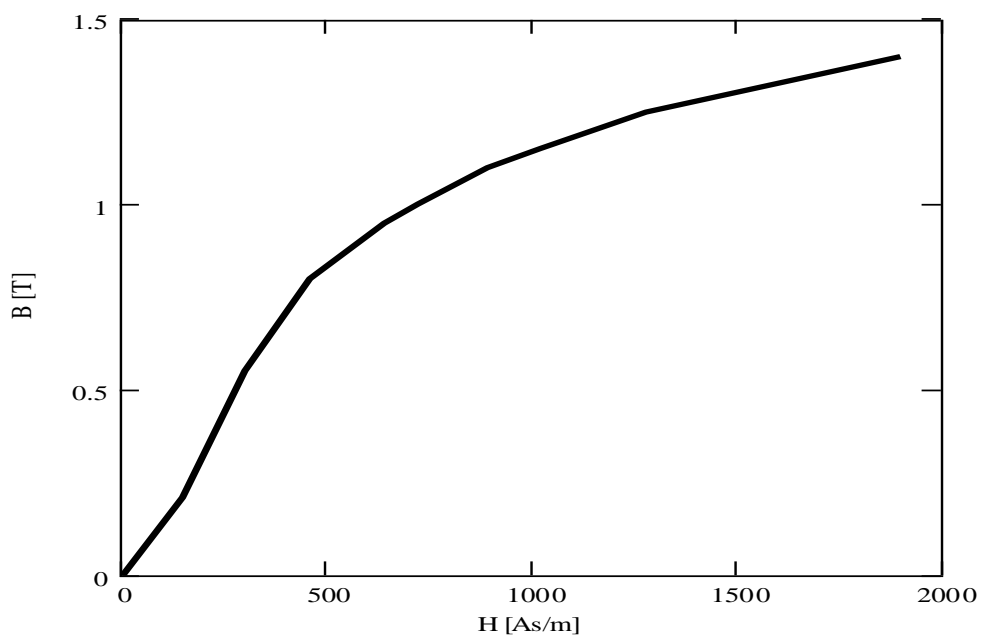
Figura 20 - Tipica curva di magnetizzazione B-H di un "ferro" commerciale usato per realizzare lo schermo.
