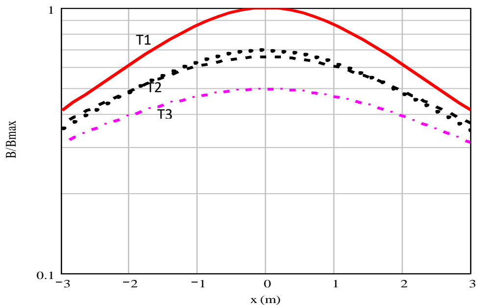
Figura 21 - Profilo laterale del flusso di induzione magnetica (in p.u.) generato da linee in cavo aventi tipiche configurazioni geometriche (i.e., T1, T2, T3 and T4 in Figura 17).
