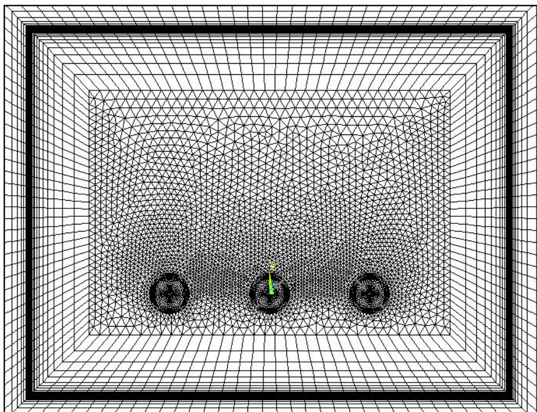
Figura 19 - Particolare della mesh generata mediante ANSYS nella regione circostante i conduttori ed in prossimità degli schermi piani.
