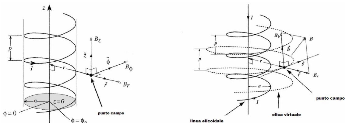
Figura 23 - Componenti del campo magnetico in coordinate cilindriche
