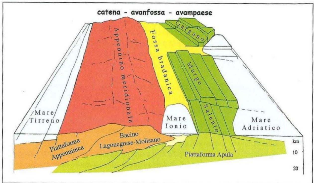
Schema geologico tridimensionale dell'Italia meridionale (da Funicello et al., 1991)
