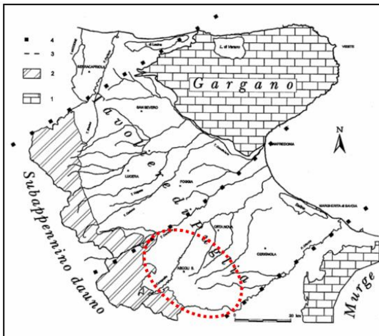
Inquadramento geologico-territoriale della Capitanata. 1) Calcarei della Piattaforma Apula; 2) Flysch del subappennino dauno; 3) limiti tra i settori: settentrionale, centrale e meridionale del Tavoliere [da Caldara & Pennetta, 1993]
