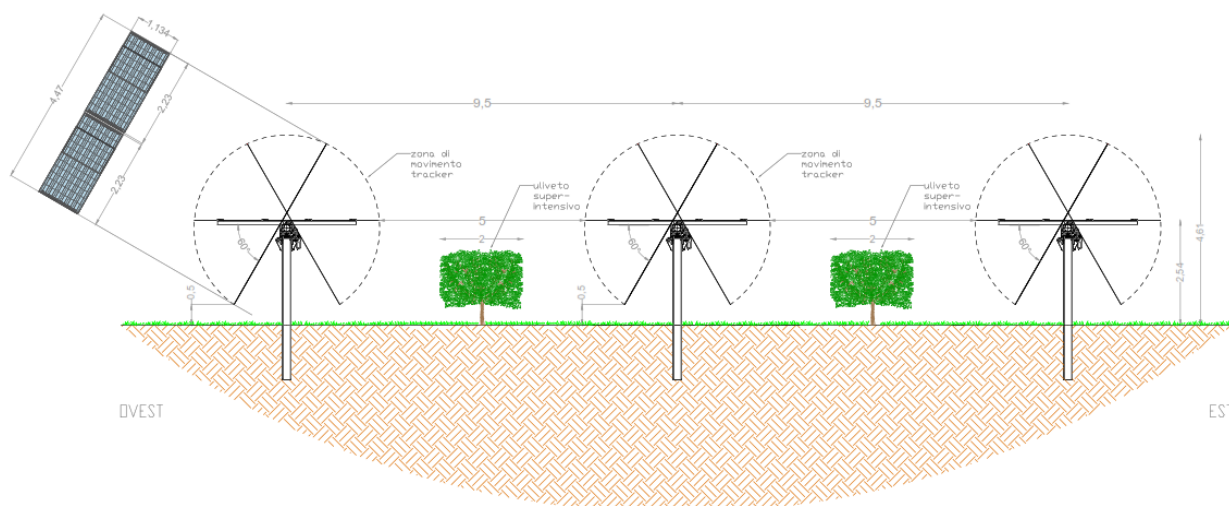
Fig. 2 Sistema Agro-fotovoltaico
