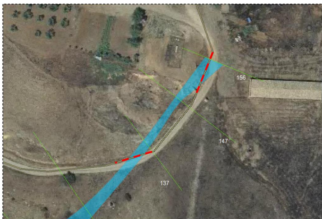
Fig. 14 Area "E Nord". Particolare del tratto di cavidotto a realizzarsi con tecnica T.O.C
