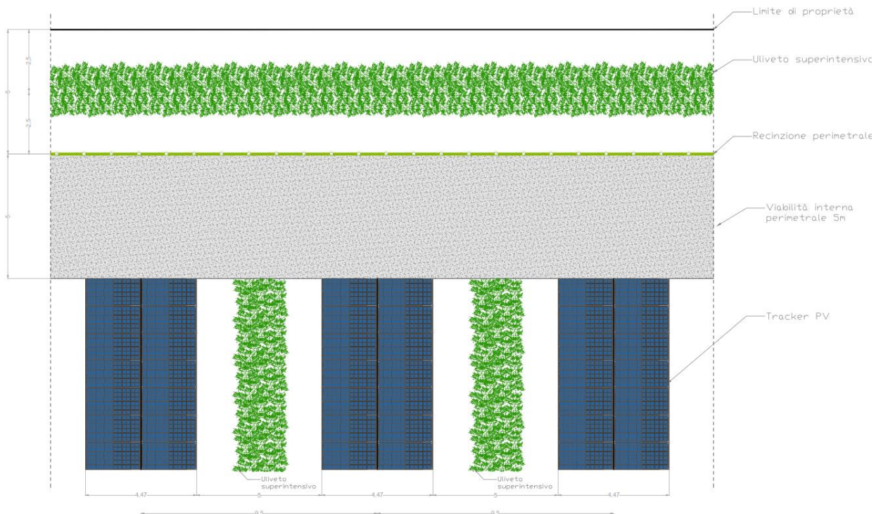
Fig. 8 Esempio di sistemazione dell'oliveto super intensivo all'interno dell'impianto fotovoltaico
