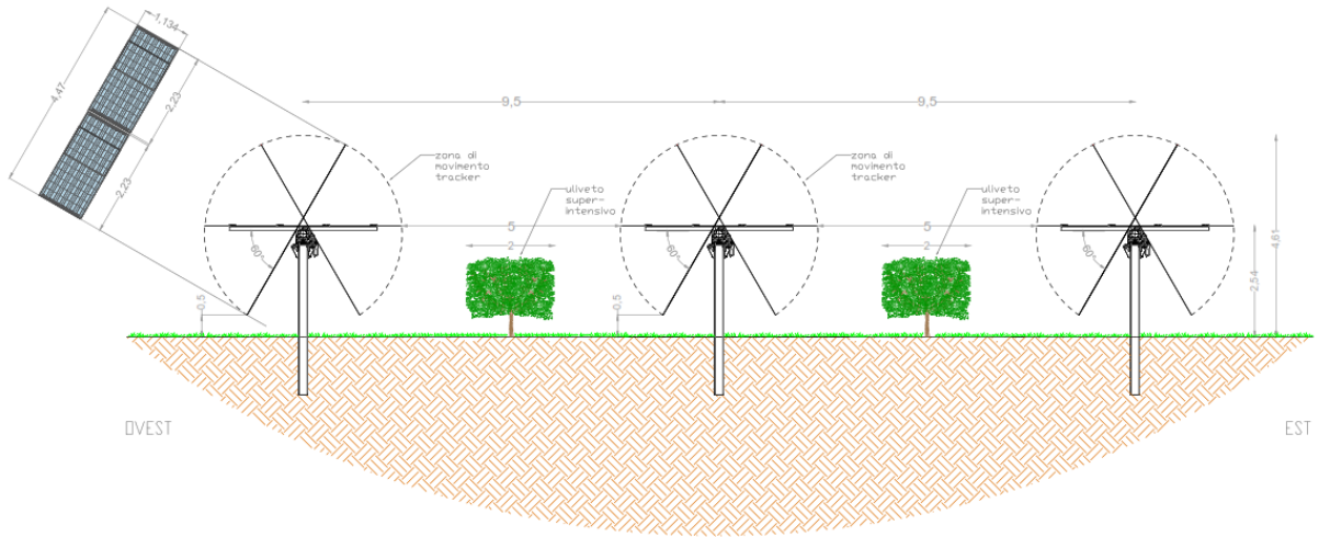
Figura 2-1: Sistema Agro-fotovoltaico
