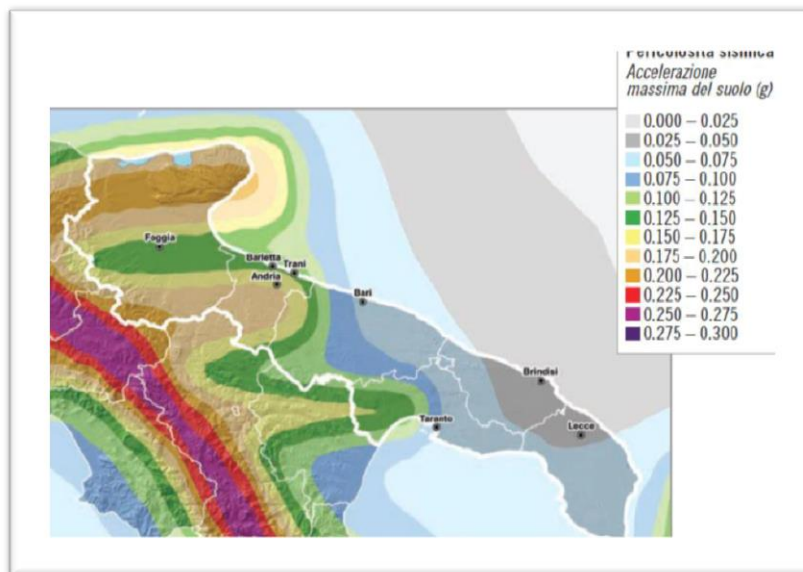
Figura 3-59: Pericolosità sismica Puglia
