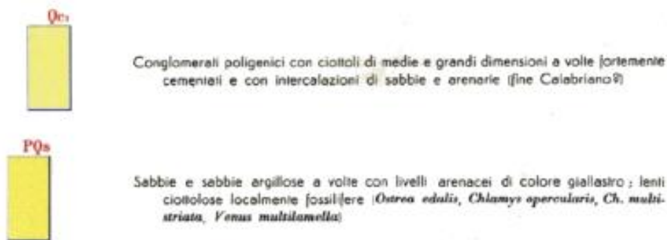
Figura 5-3: Stralcio Carta Geologica d'Italia, Foglio 175 "Cerignola"
