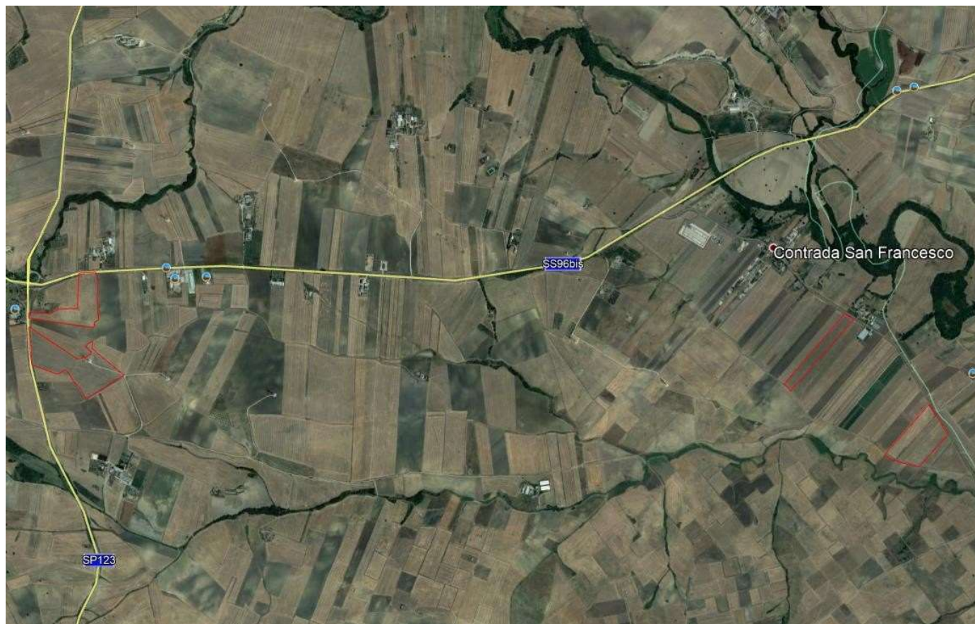
Aree di progetto dell'impianto fotovoltaico su ortofoto.
