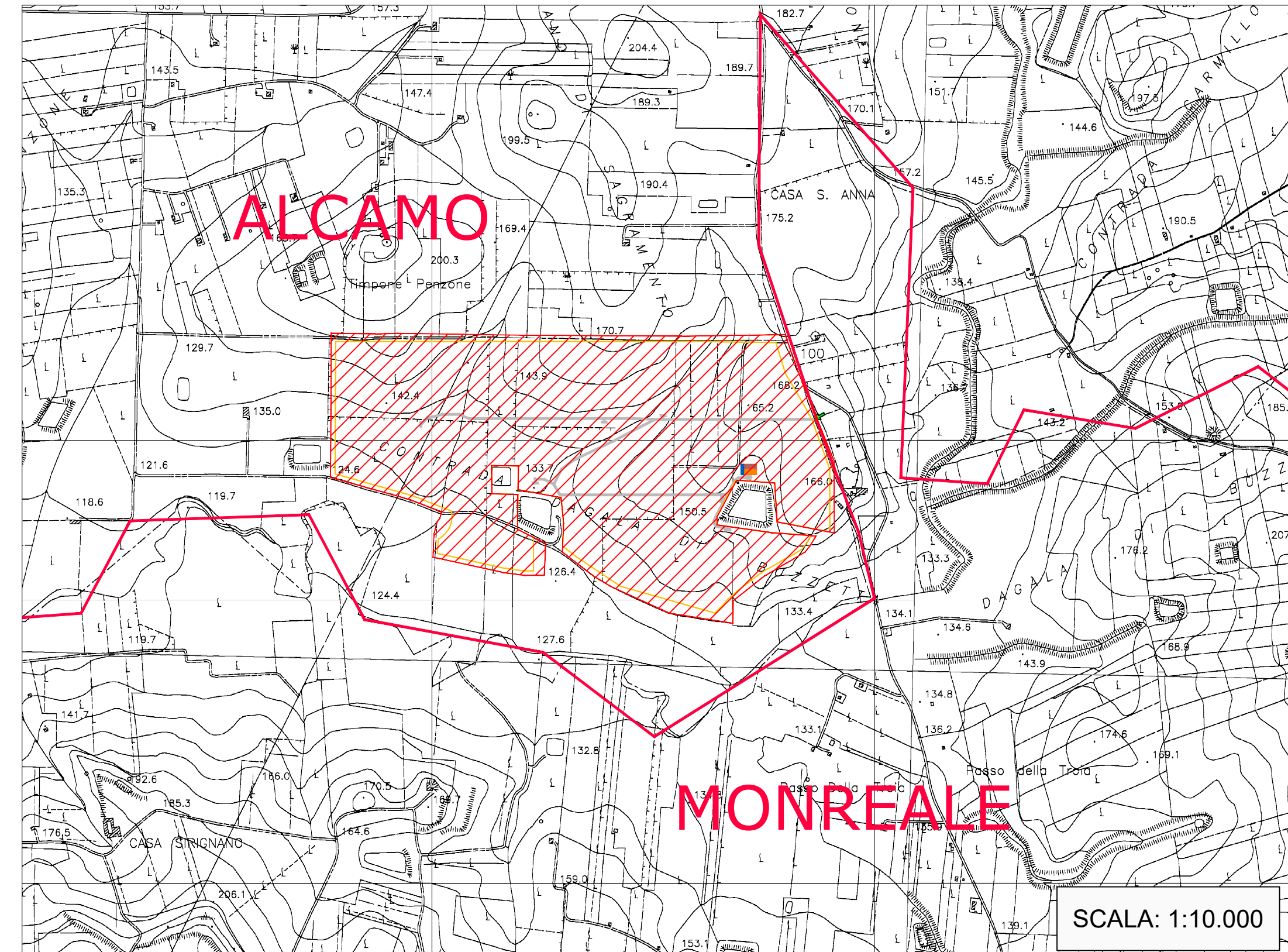
LEGENDA PLANIMETRIE AREE DI CANTIERIZZAZIONE
