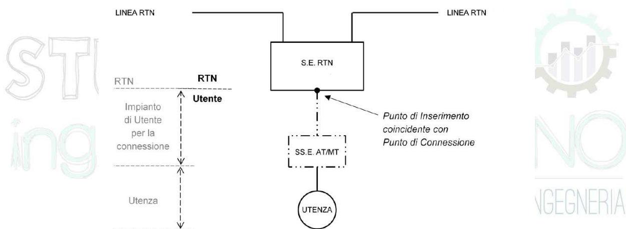
fig. 3 - INSERIMENTO IN ANTENNA
