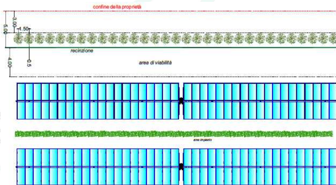
Figura 2-2: Soluzione Agro-Solare: barriera verde perimetrale, viabilità interna, tracker e componente agronomica: Mandorleto Intensivo
