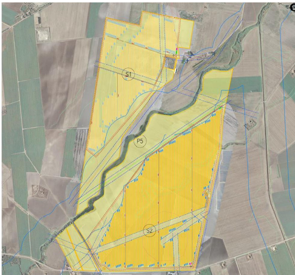
Figura 2.1: Localizzazione dell'area di intervento, in giallo l'area contrattualizzata in rosso la recinzione dell'impianto
