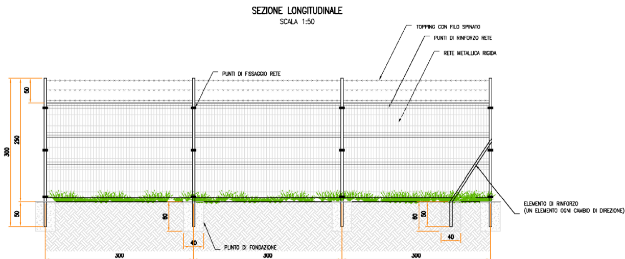
Figura 5.1: Tipico recinzione
