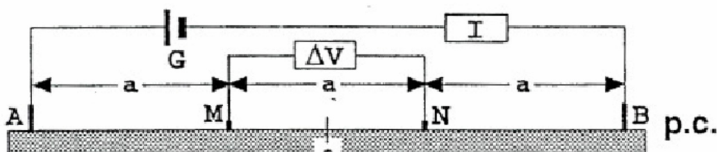
Figura 6 – Dispositivo Wenner -
