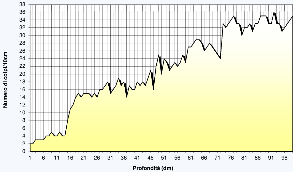
PROVA PENETROMETRICA 23
