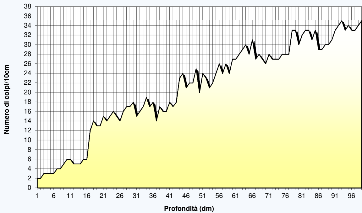
PROVA PENETROMETRICA 24
