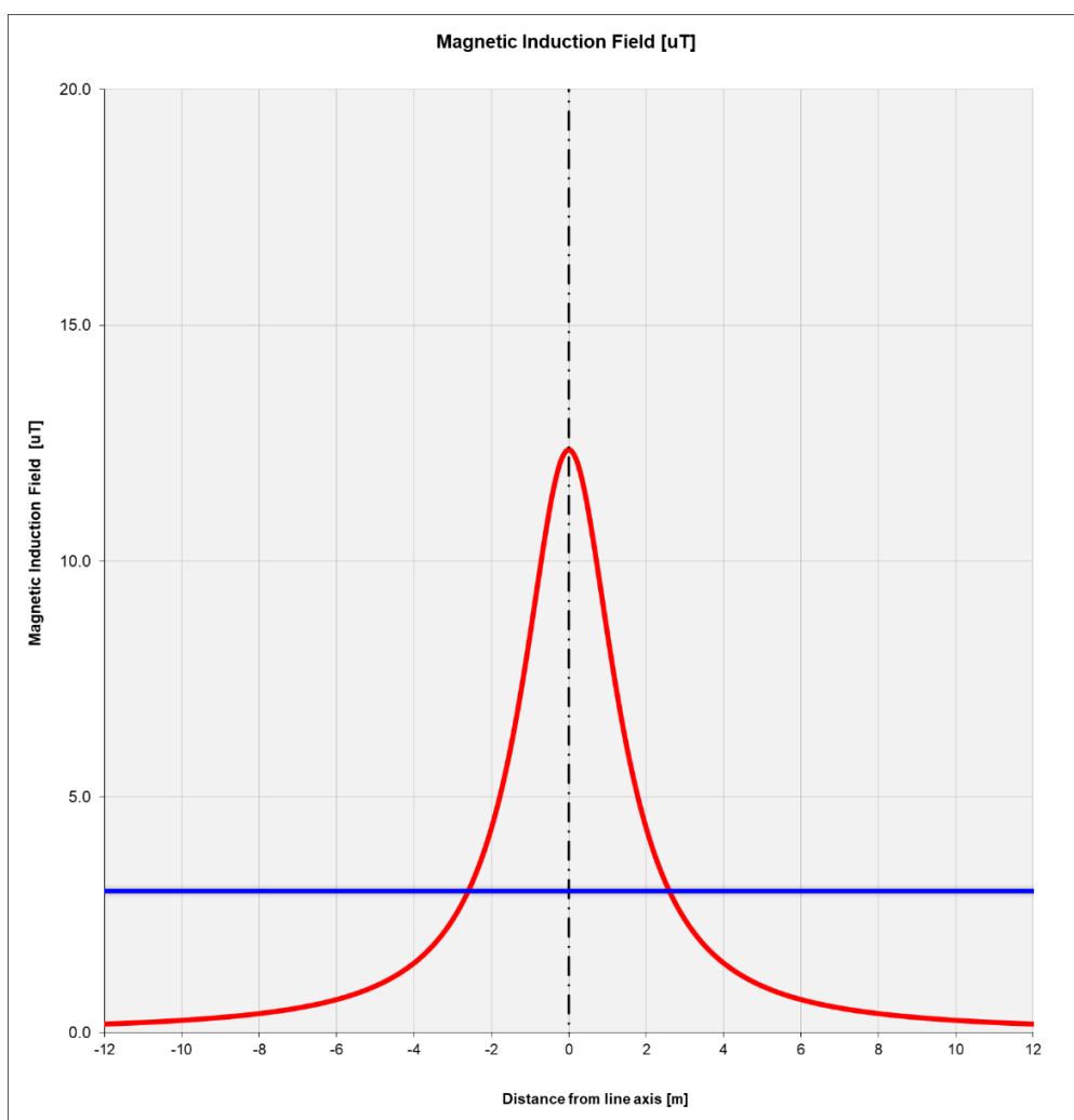
Figura 3: Andamento dell'induzione magnetica prodotta dalla linea in cavo di collegamento con la SSEU
