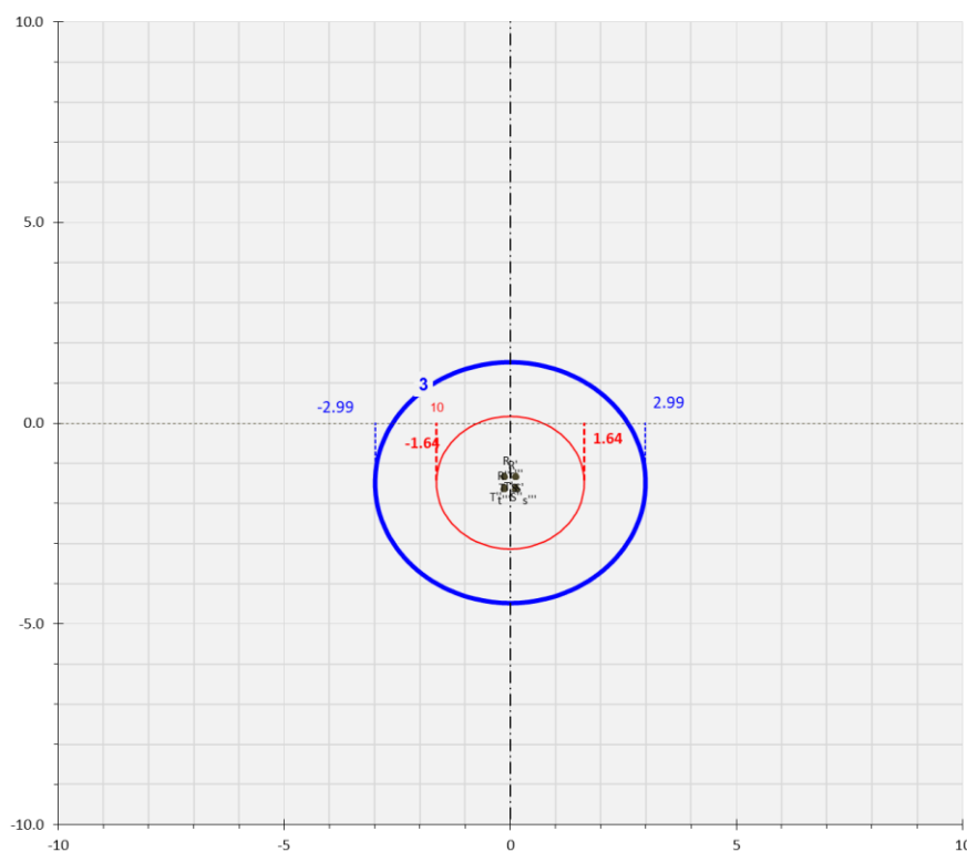
Figura 4: Curve di equilivello per il campo di induzione magnetica generato dalla linea MT di collegamento con la SSEU
