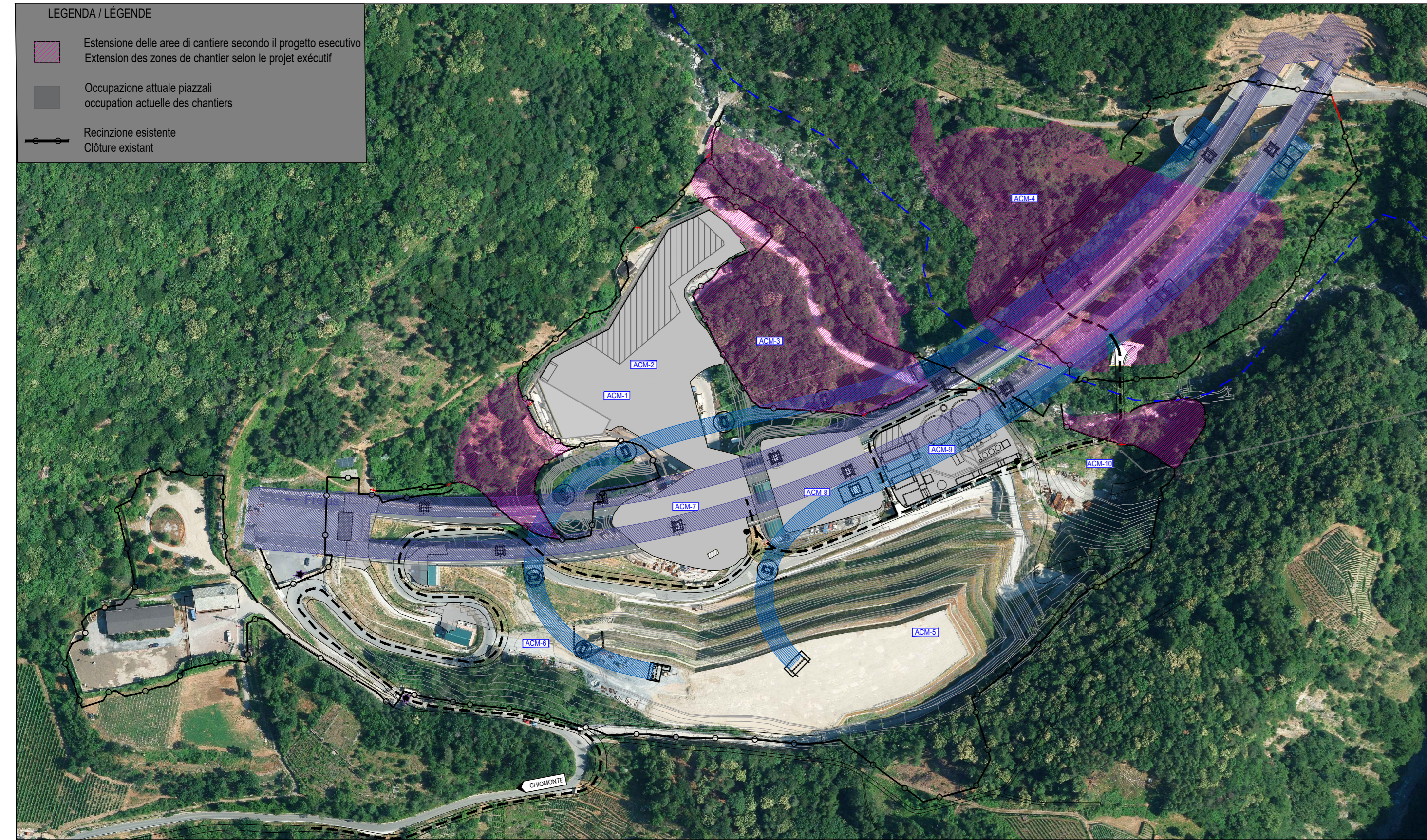
PLANIMETRIA / VUE EN PLAN - Scala 1:1000 / Echelle 1:1000
