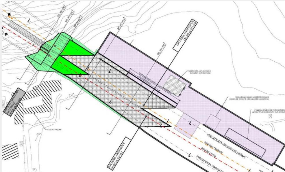
Planimetria imbocco est tunnel di base
