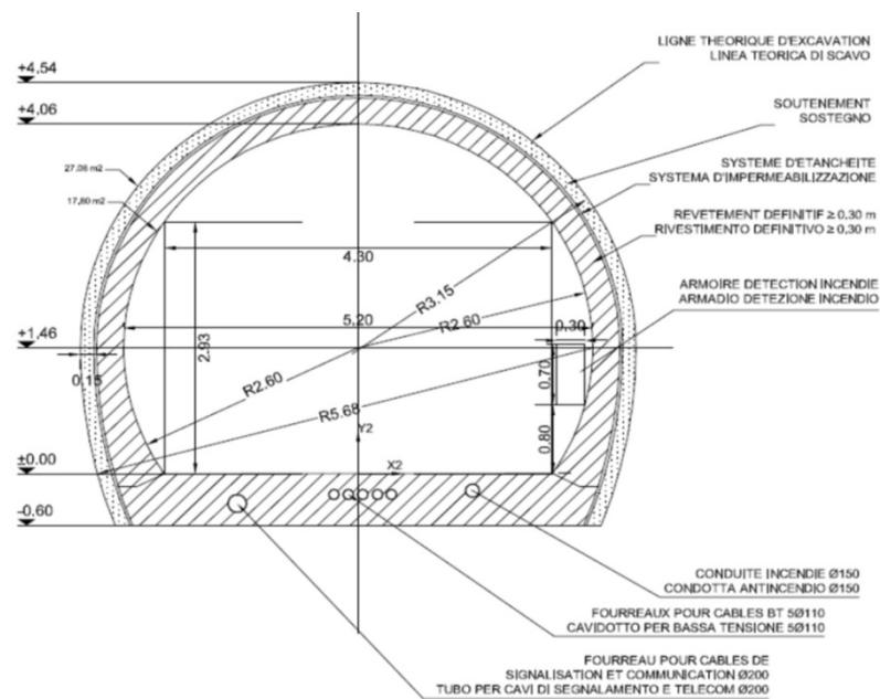
Sezione corrente ramo di collegamento
