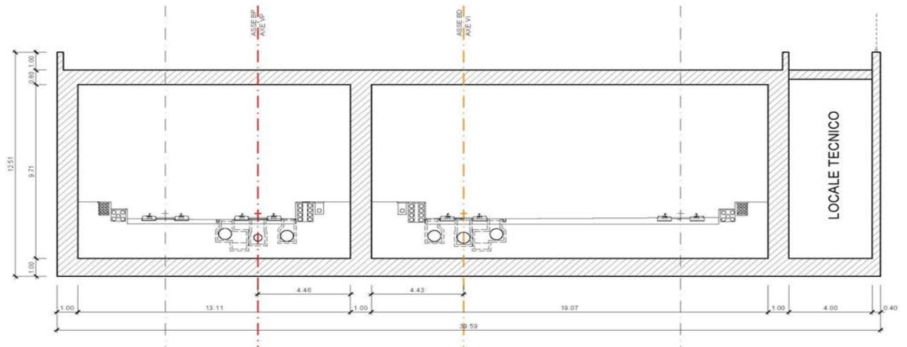
Sezione Tipo Galleria Artificiale Da Pk 61+105 A Pk 61+182 Binario Pari
