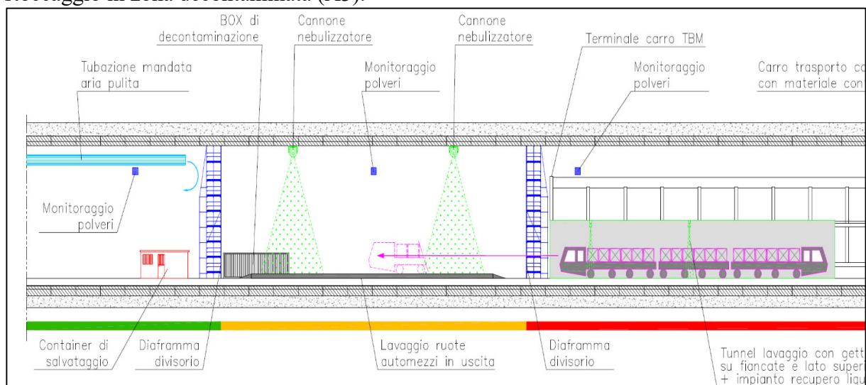
Figura 18 – Trasporto dei cassoni e lavaggio dei mezzi
