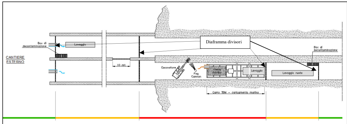
Figura 19 – Scavo con martello demolitore nella zona di imbocco
