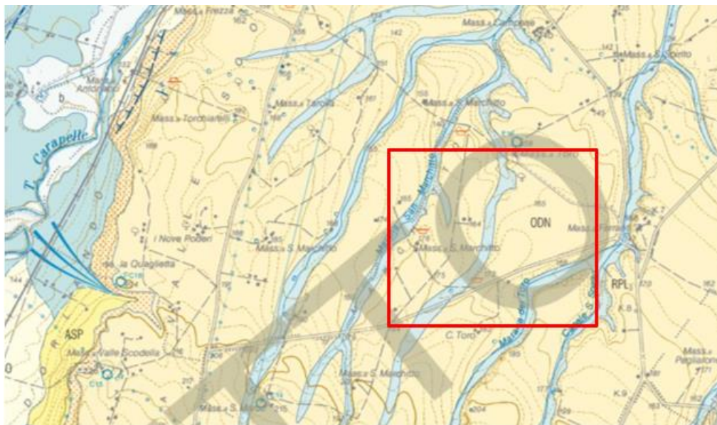
Figura 9 – Estratto della Carta Geologica Foglio 421 Ascoli Satriano - Nel riquadro le aree di insediamento dell'impianto fotovoltaico.
