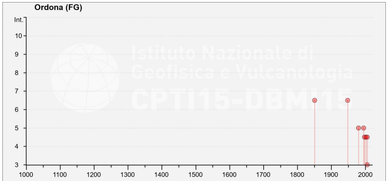
Figura 20 – Storia sismica del Comune di Ordona [41.315, 15.628] – https://emidius.mi.ingv.it/CPT115-DBMI15_v1.5/query_place/
