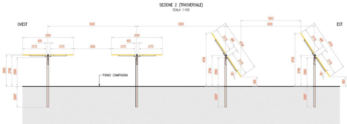
Particolare strutture sostegno moduli e distanze di campo
