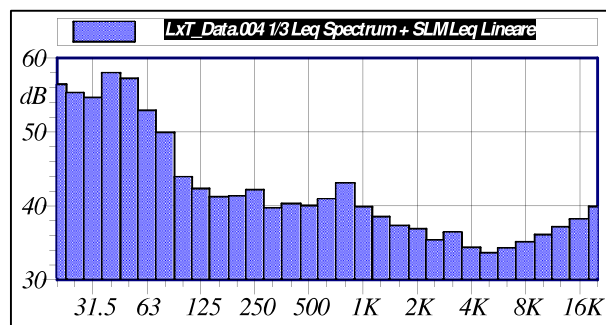
SPETTRO MEDIO
