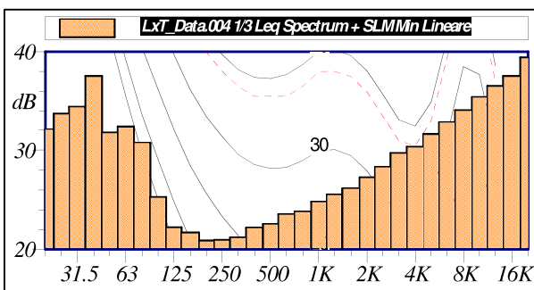
SPETTRO MINIMI
