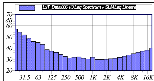
SPETTRO MEDIO
