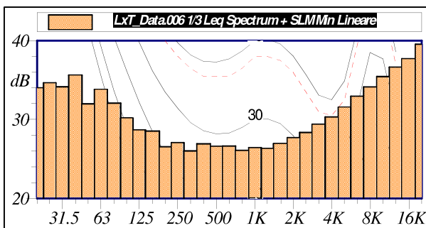
SPETTRO MINIMI
