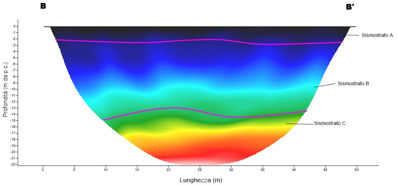
Fig. 8 – Interpretazione sezione tomografica del profilo BB'
