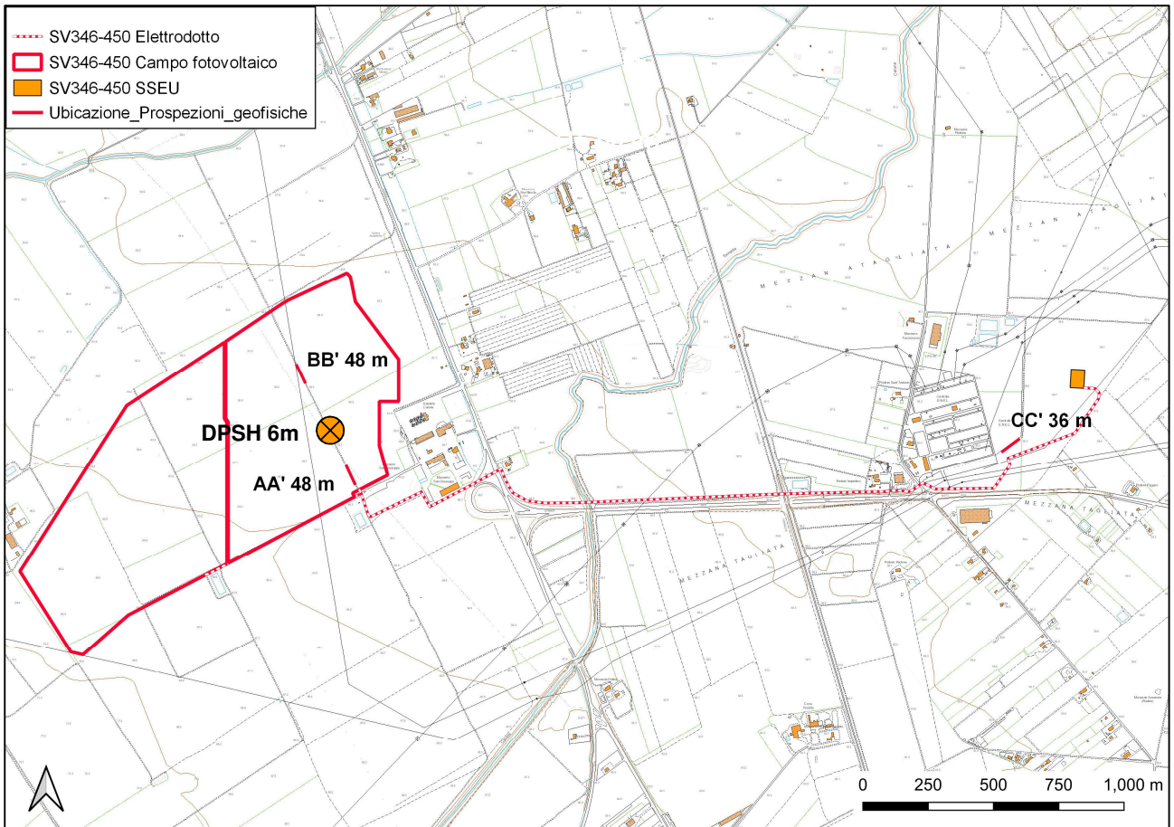
Figura 6 – Ubicazione degli stendimenti geofisici e della prova penetrometrica DPSH
