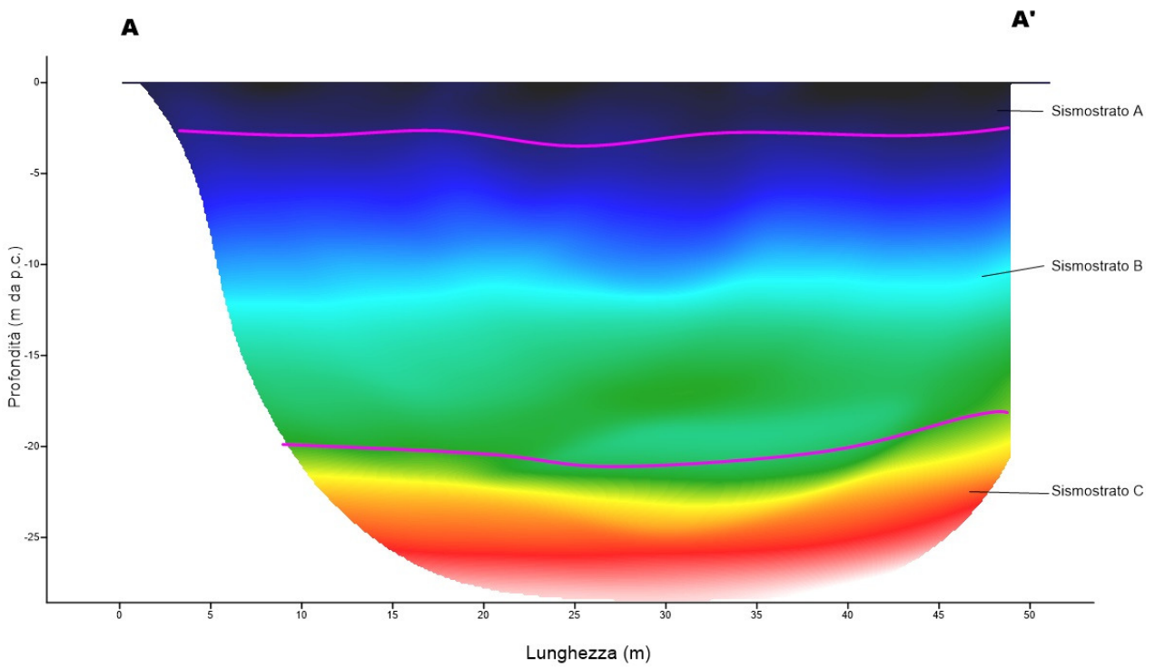
Fig. 7 – Interpretazione sezione tomografica del profilo AA'
