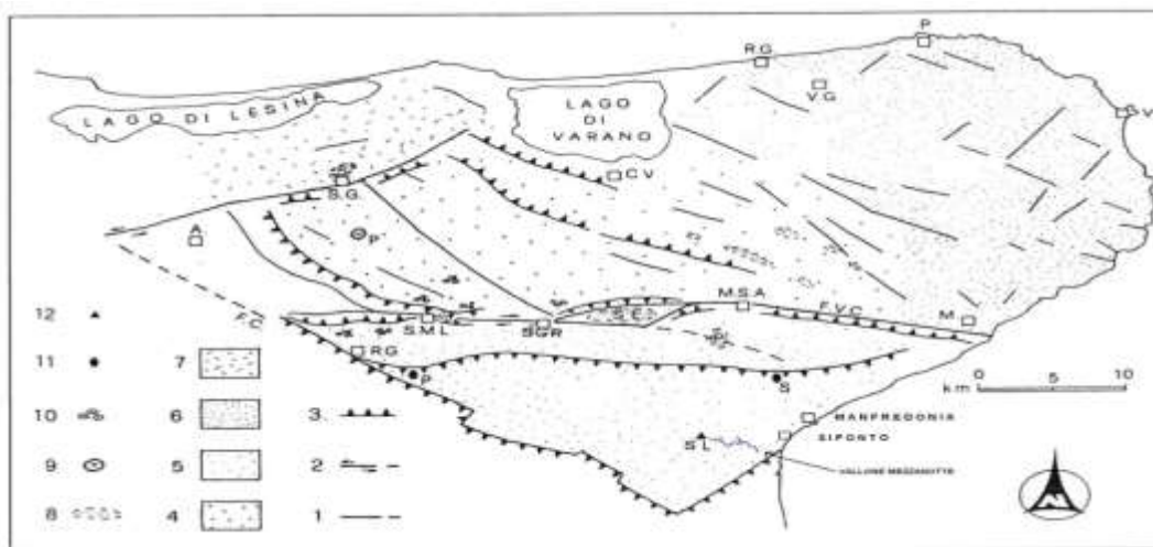
Fig.– Schema morfotettonico generale del promontorio del Gargano (da Caldara M. & Palmentola G.,1993, modificata). Legenda: 1= faglia, 2= faglia trascorrente, 3= scarpata di linea di faglia, 4= altopiano centrale carsico, 5= regione dei terrazzi meridionali, 6= versante orientale di modellamento torrentizio, 7= regione dei terrazzi nord-occidentali, 8= polye, 9= dolina,10= campi di doline, 11= grotta, 12 = centri abitati con abbreviazione.
