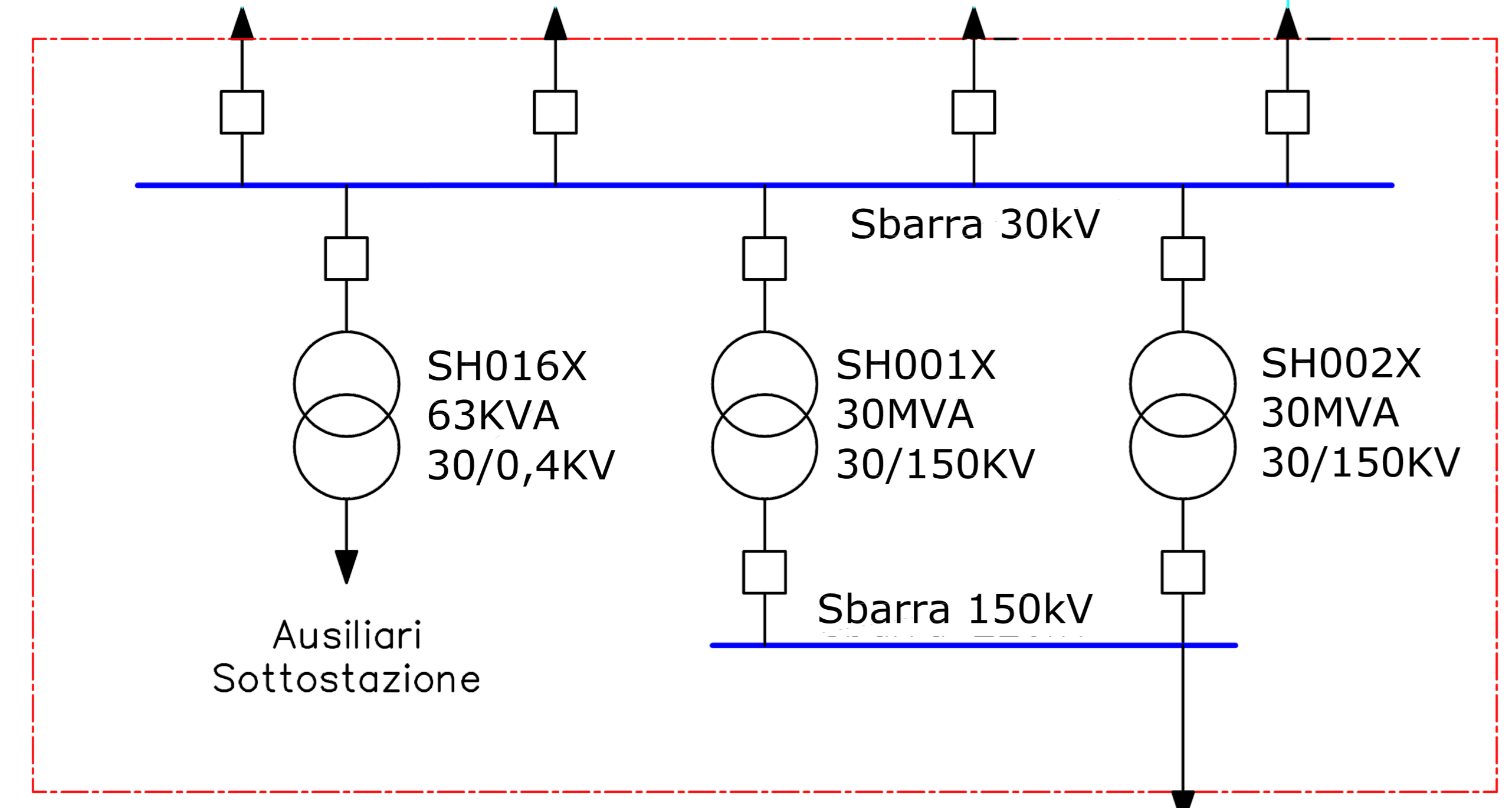
Sottostazione di Trasformazione MT/AT
