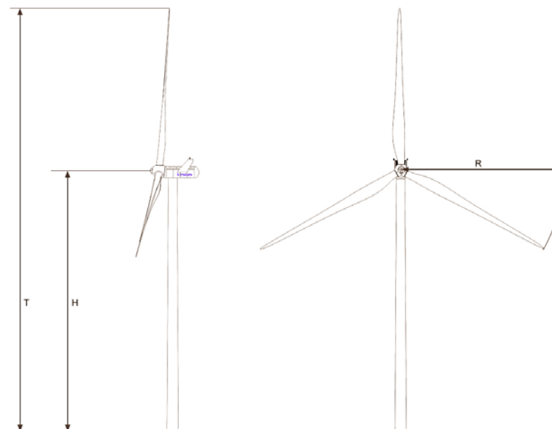
Figura 3.1.a.: Schema Aerogeneratore Vestas V112-3MW
