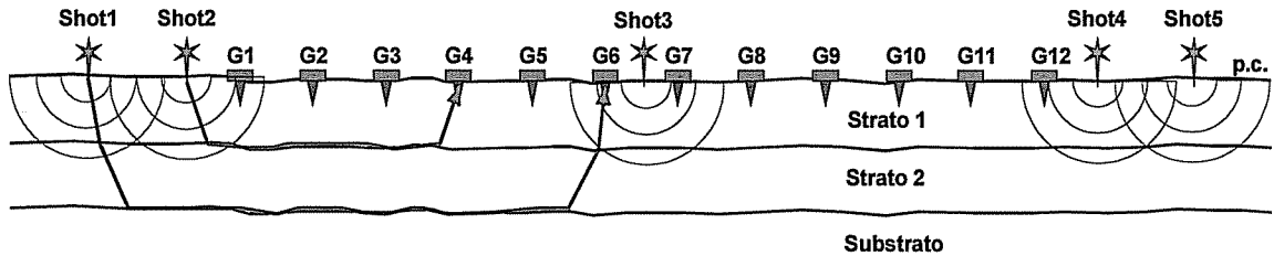
Fig. 1 - geometria dello stendimento.
