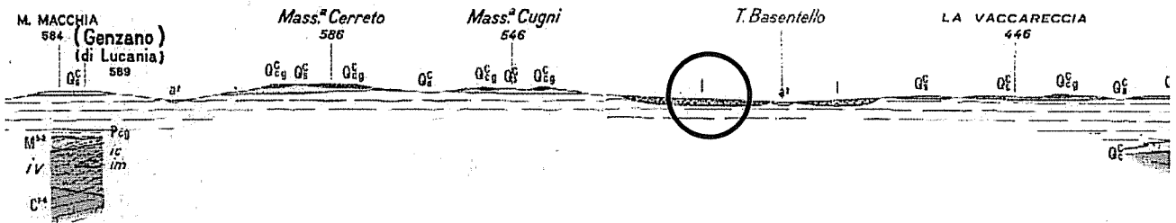
L'area oggetto di studio è situata nell'Avanfossa Bradanica.
