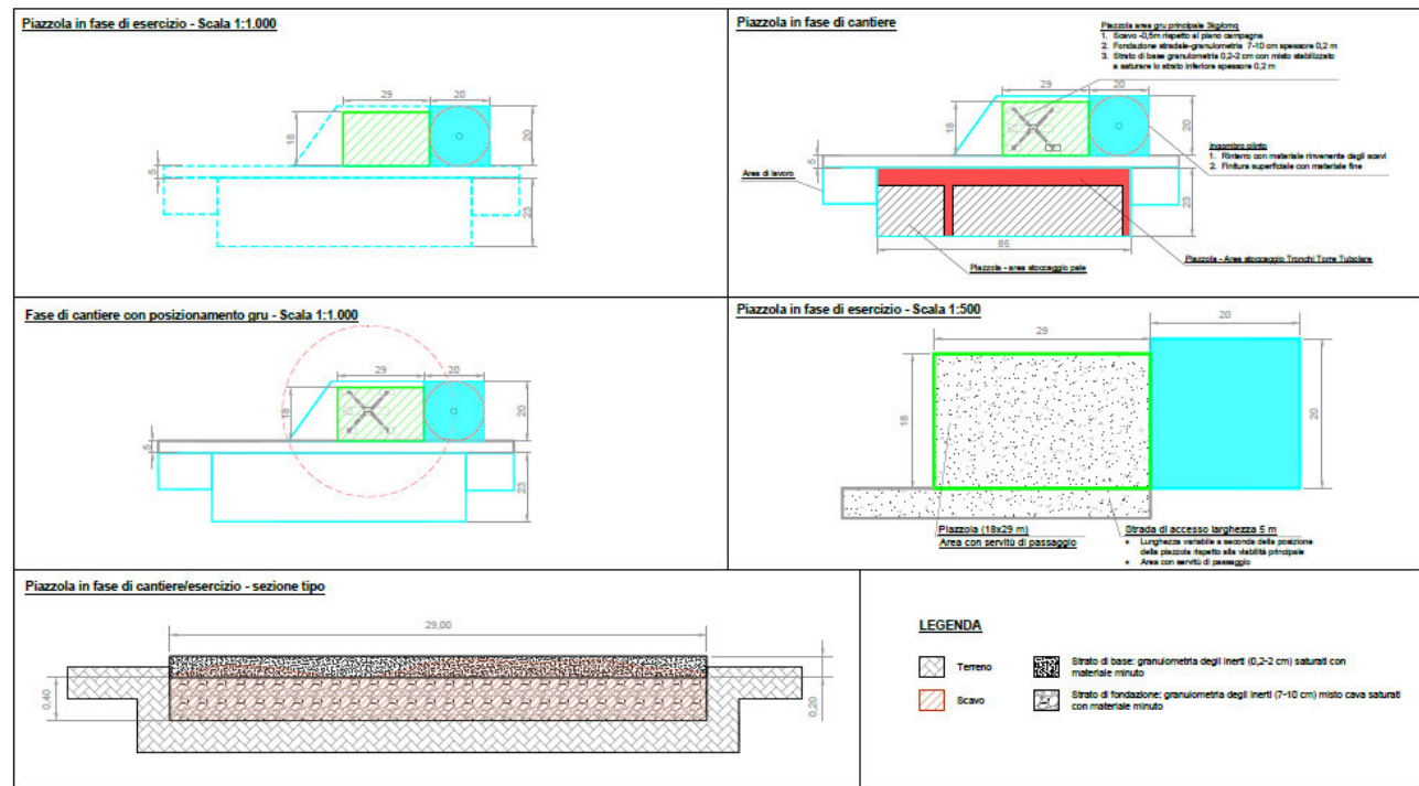
Figura 7 | Piazzola di assemblaggio aerogeneratore
