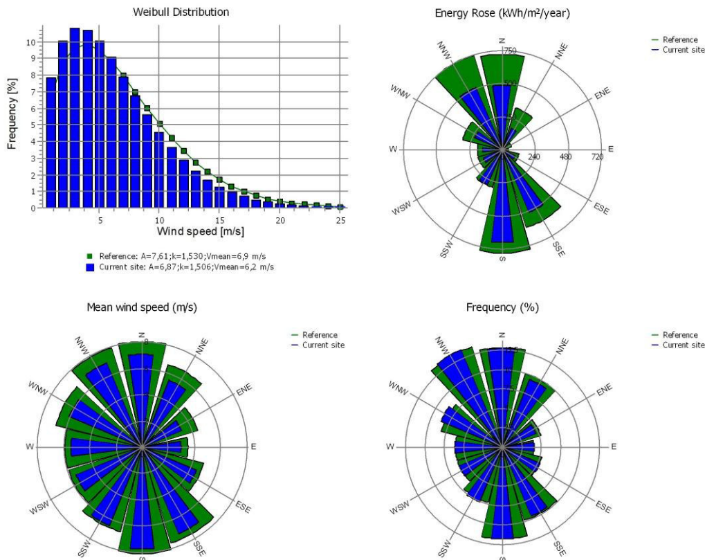
Figura 6 | Dati vento processati
