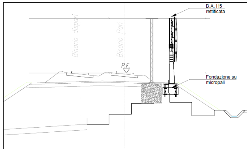
Barriera acustica su basamento in cls
