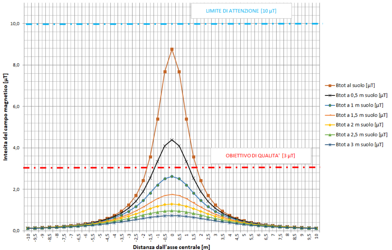
Fig. n°4 Intensità del campo magnetico al variare dell'altezza dal suolo del tratto LB di cavidotto
