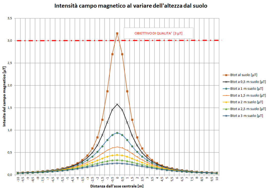
Fig. n°3 Intensità del campo magnetico al variare dell'altezza dal suolo del tratto LB di cavidotto
