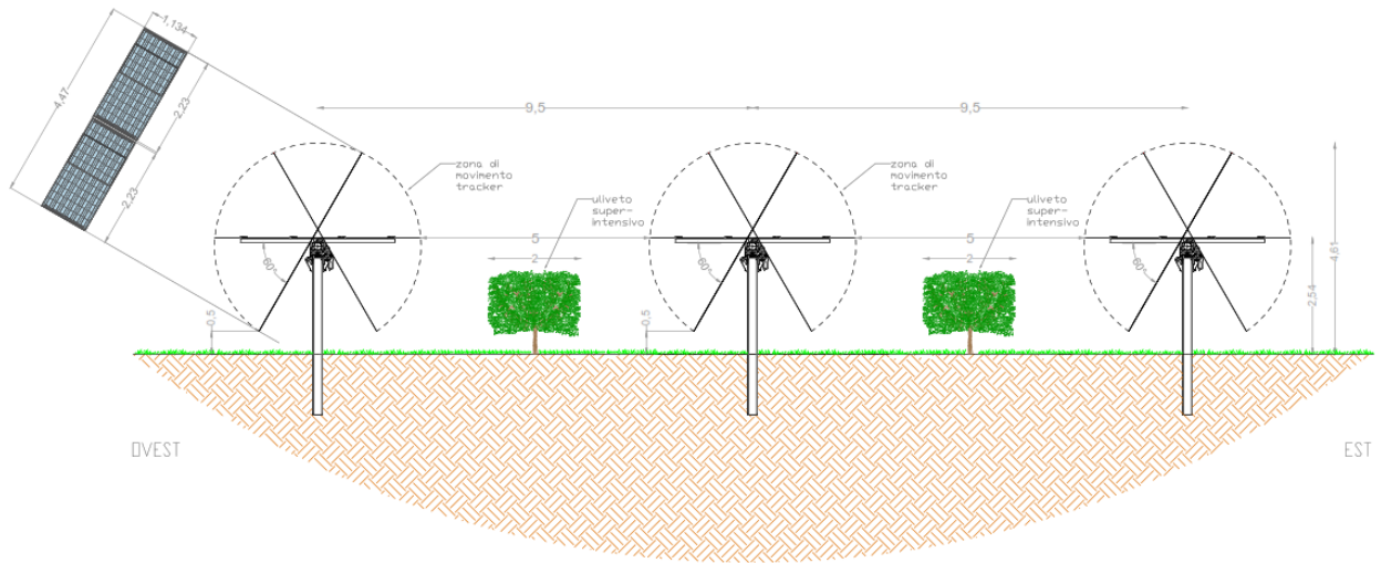
Fig. n°18 Pitch dei tracker
