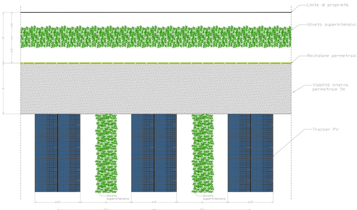
Fig. 4 Esempio di sistemazione dell'oliveto super intensivo all'interno dell'impianto fotovoltaico
