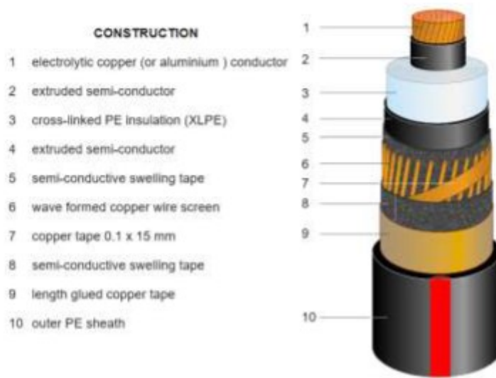
Fig. 19 Stratigrafia cavo AT
