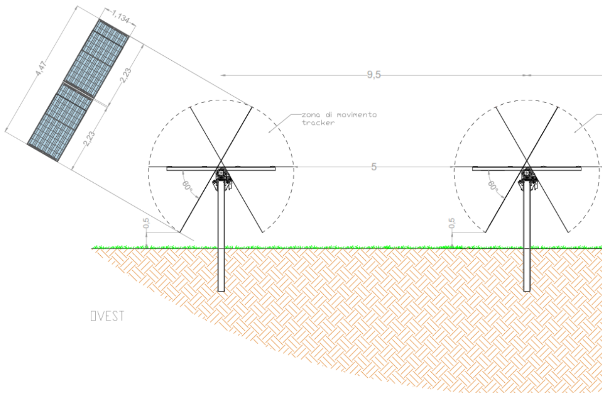
Fig. n°17 Angolo rotazione del tracker
