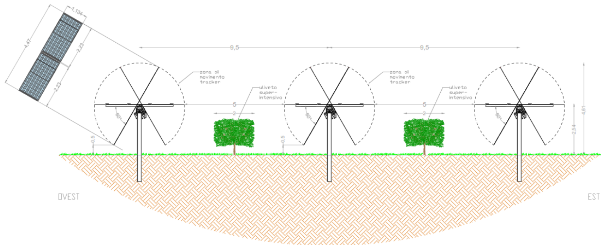
Fig. 1 Sistema Agro-fotovoltaico
