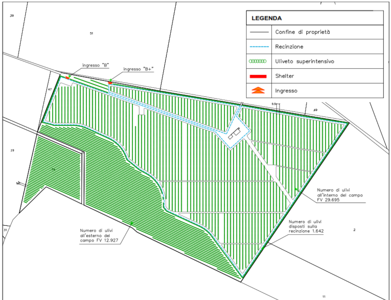
Fig.5 Impianto agro-fotovoltaico blocco "B" - aree destinate all'agricoltura e misure mitigative
