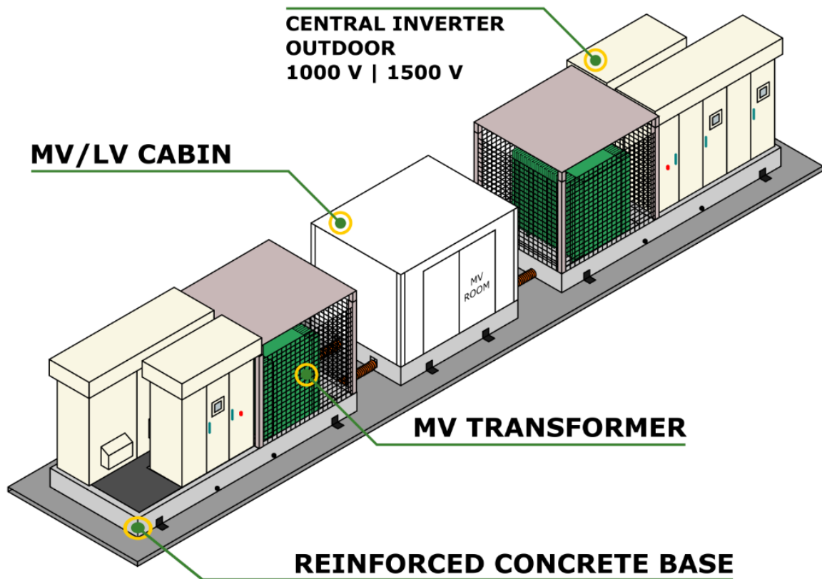
Fig. n°14 Power Skid
