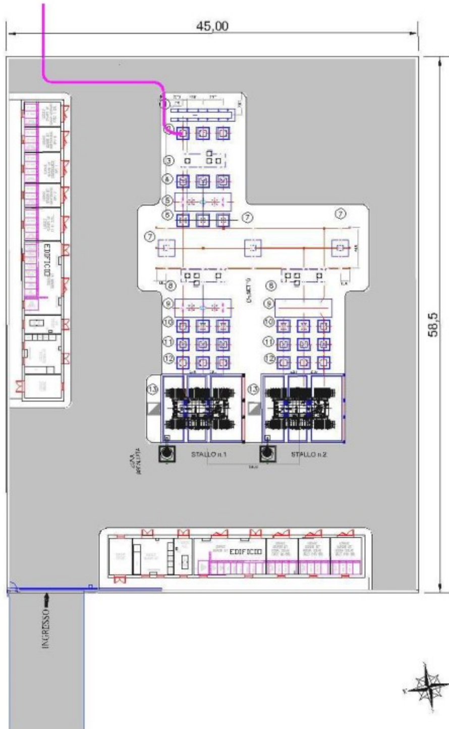
Fig. 10 Planimetria sottostazione utente
