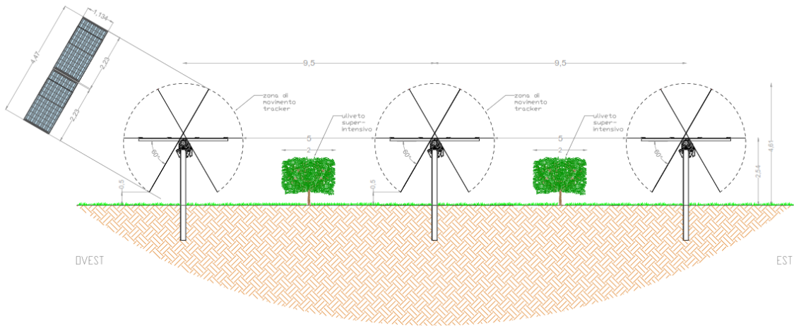
Figura 4-3: Schema d'impianto dell'uliveto super intensivo tra i pannelli fotovoltaico – vista in sezione
