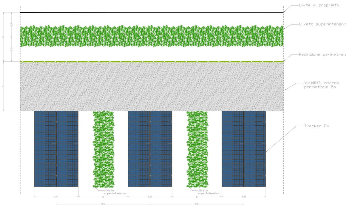
Figura 2-4: Esempio di sistemazione dell'oliveto super intensivo all'interno dell'impianto fotovoltaico
