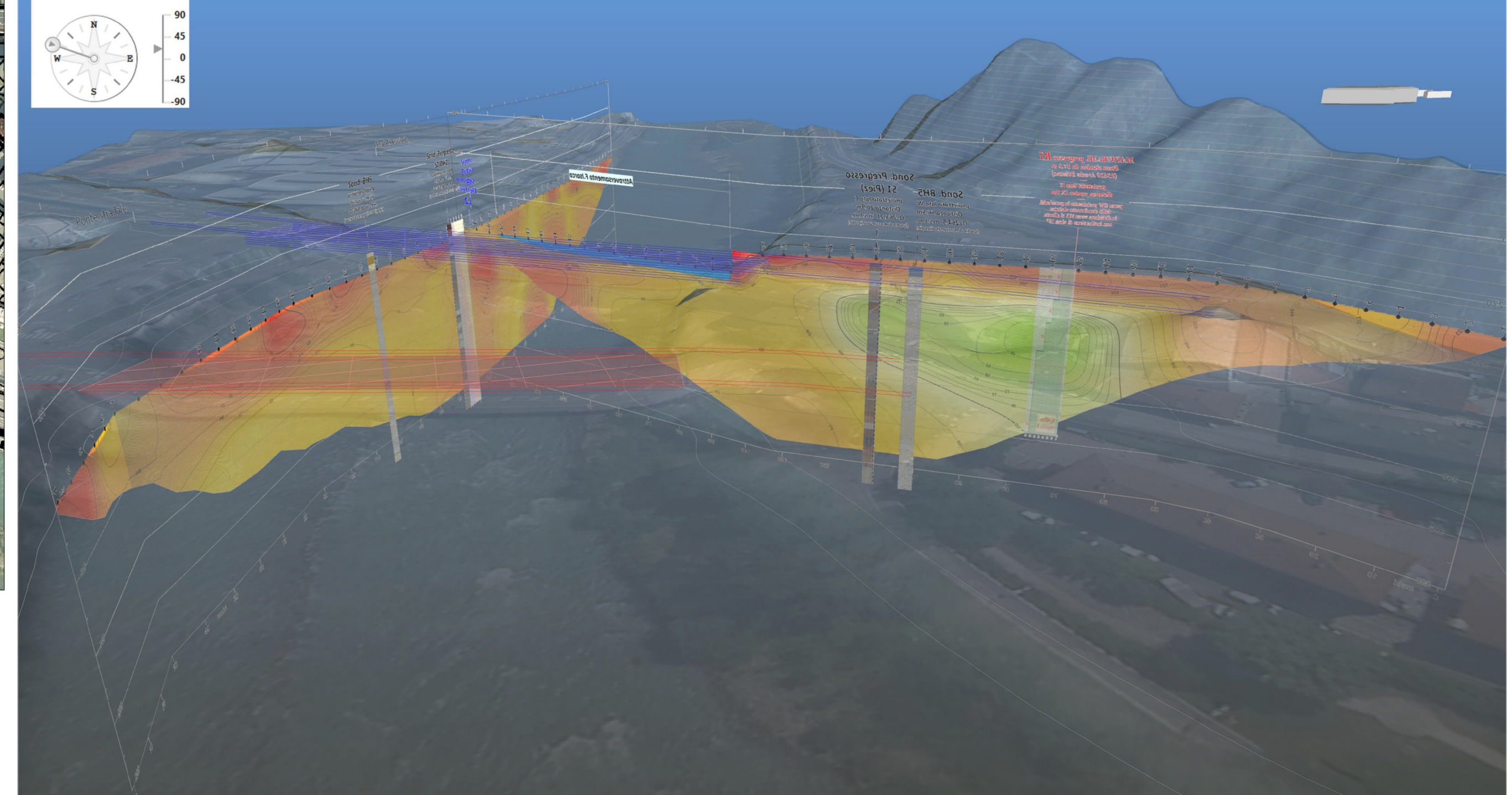
Vista 3D delle Sezioni Elettriche: L1 - attraversamento F.Isarco in prossimità del ponte ferroviario, L2 - parallela al F.Isarco
