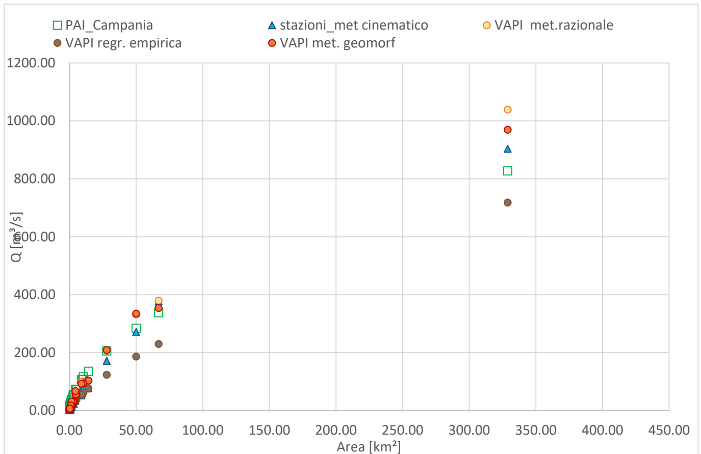
Figura 5 – Portate calcolate con i diversi metodi per i sottobacini del lotto 1A in funzione dell'area sottesa alla sezione dell'interferenza idraulica
