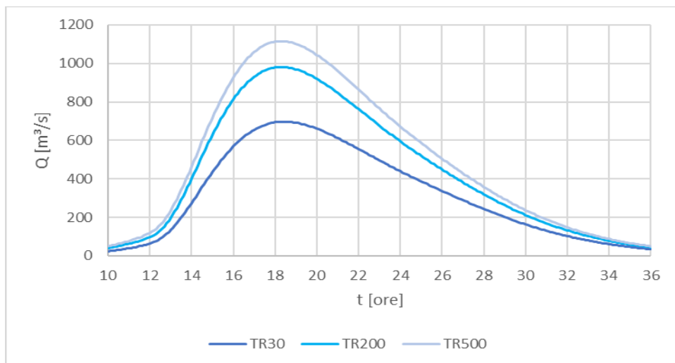
Figura 8 – Idrogrammi di piena – fiume Sele alla sezione dell’attraversamento ferroviario
