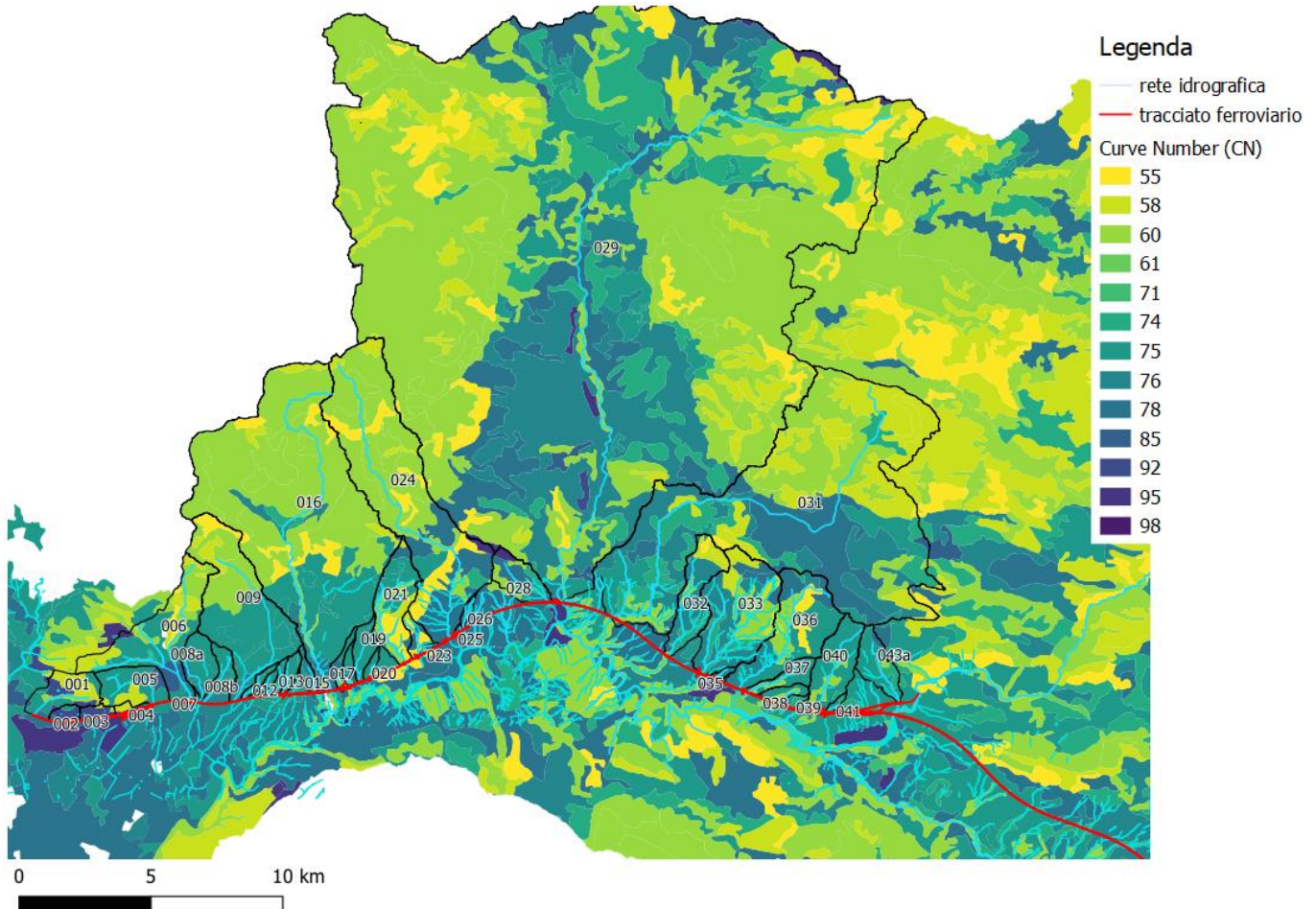
Figura 4 – Rappresentazione cartografica del CN nell'area di studio (bacini del lotto 1A)
