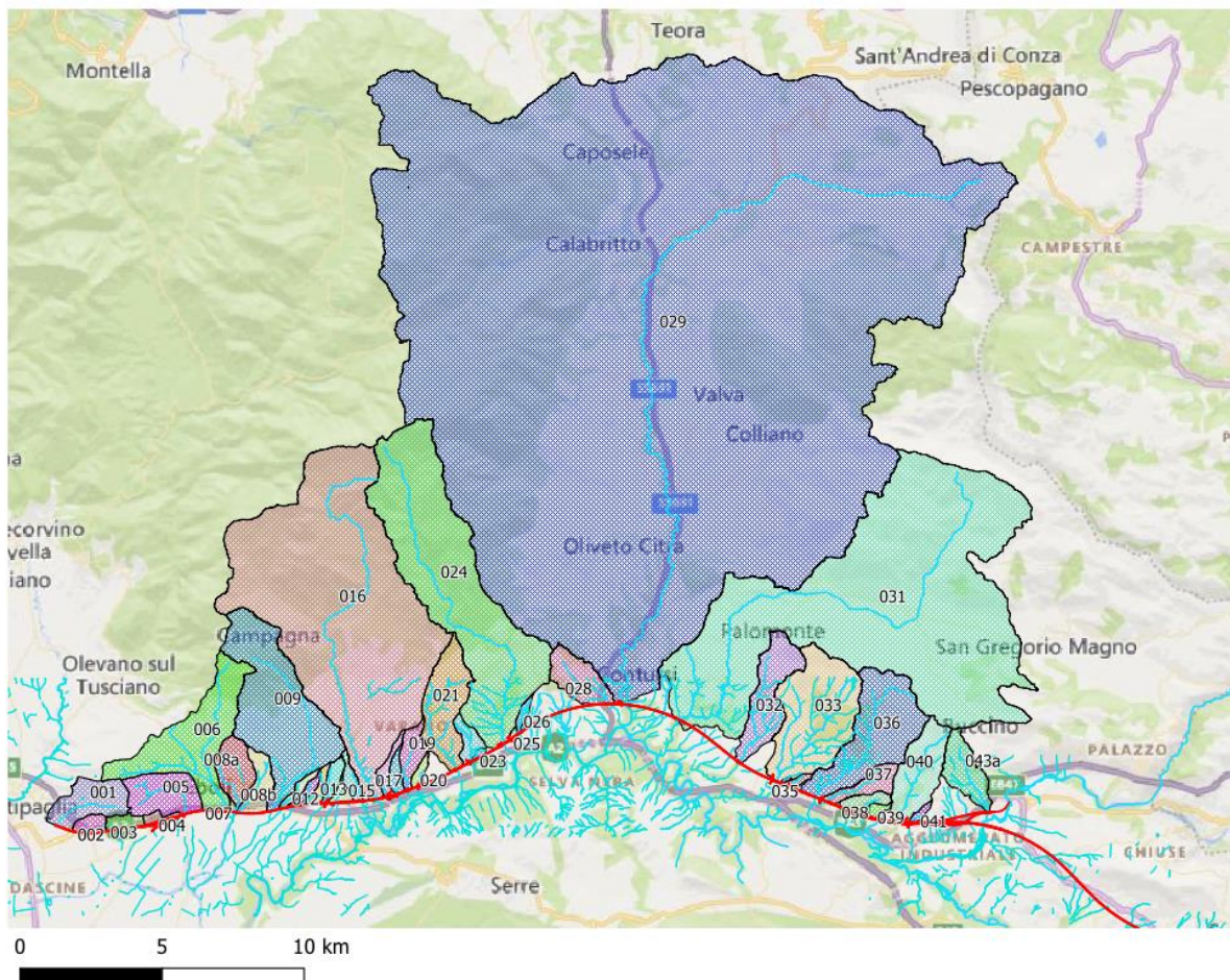
Figura 3 – Delimitazione dei bacini del lotto 1A
