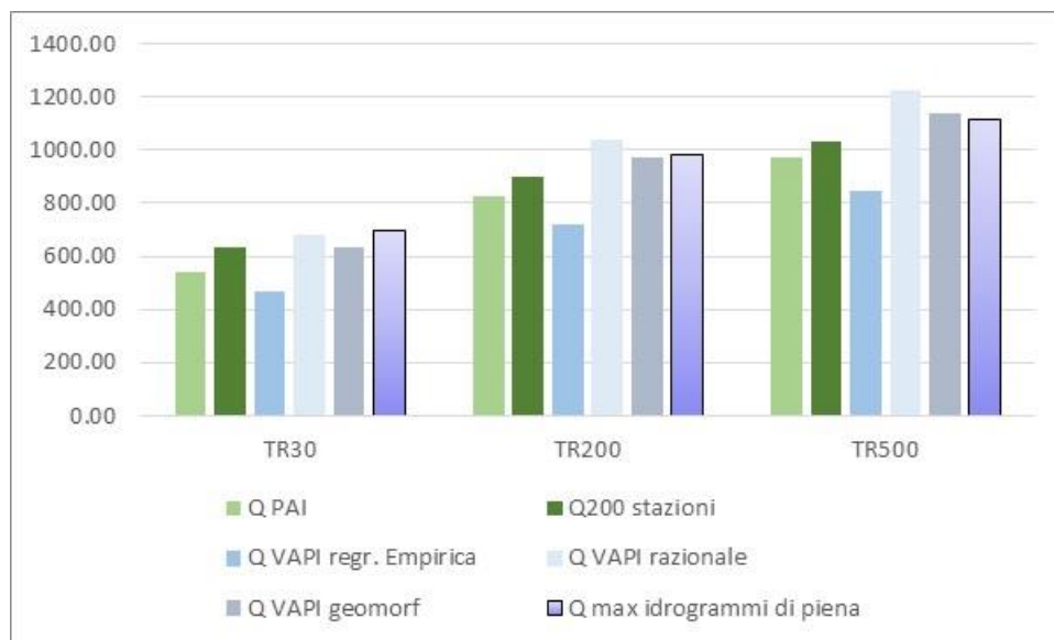
Figura 9 – Confronto delle portate al colmo ottenute con i diversi metodi (in blu sfumato quelli mediante modellazione in HEC HMS)
