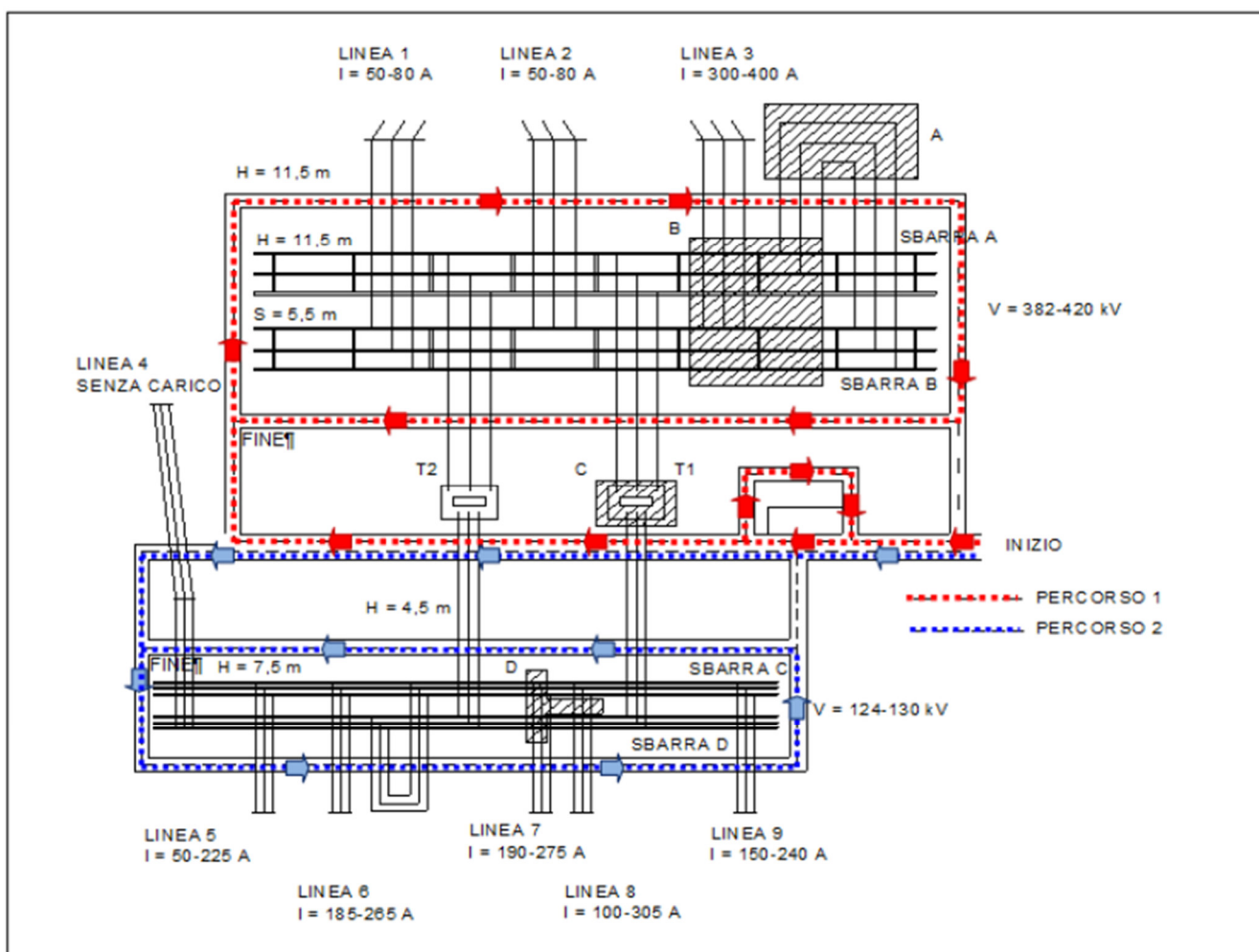
Fig. 1 – Pianta di una tipica stazione 380/150 kV: indicazione delle principali distanze fase-fase ( S ) e fase-terra ( H ) e delle variazioni delle tensioni e delle correnti durante le fasi di misurazioni di campo elettrico e magnetico
