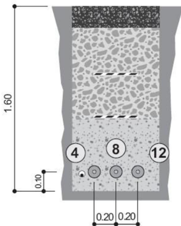
Fig. 6a – Rappresentazione di interrimento "in piano" di una semplice terna in cavo unipolare esercita a 150 kV
