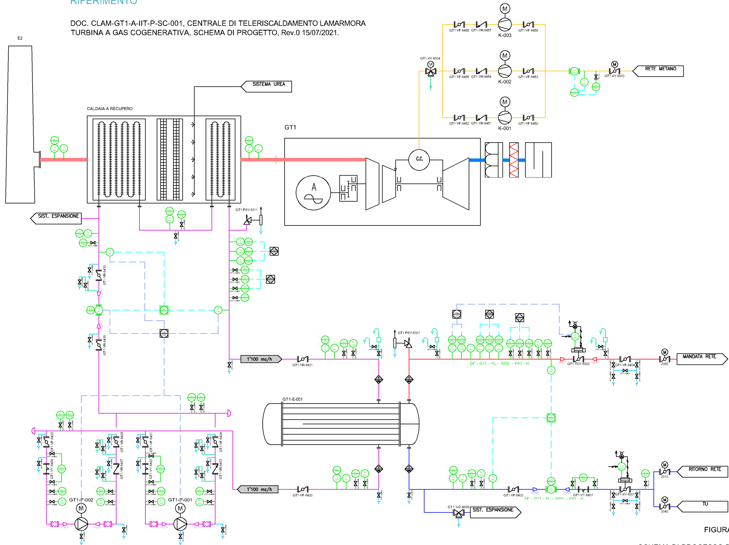
SCHEMA DI PROCESSO DEL NUOVO TURBOGAS
