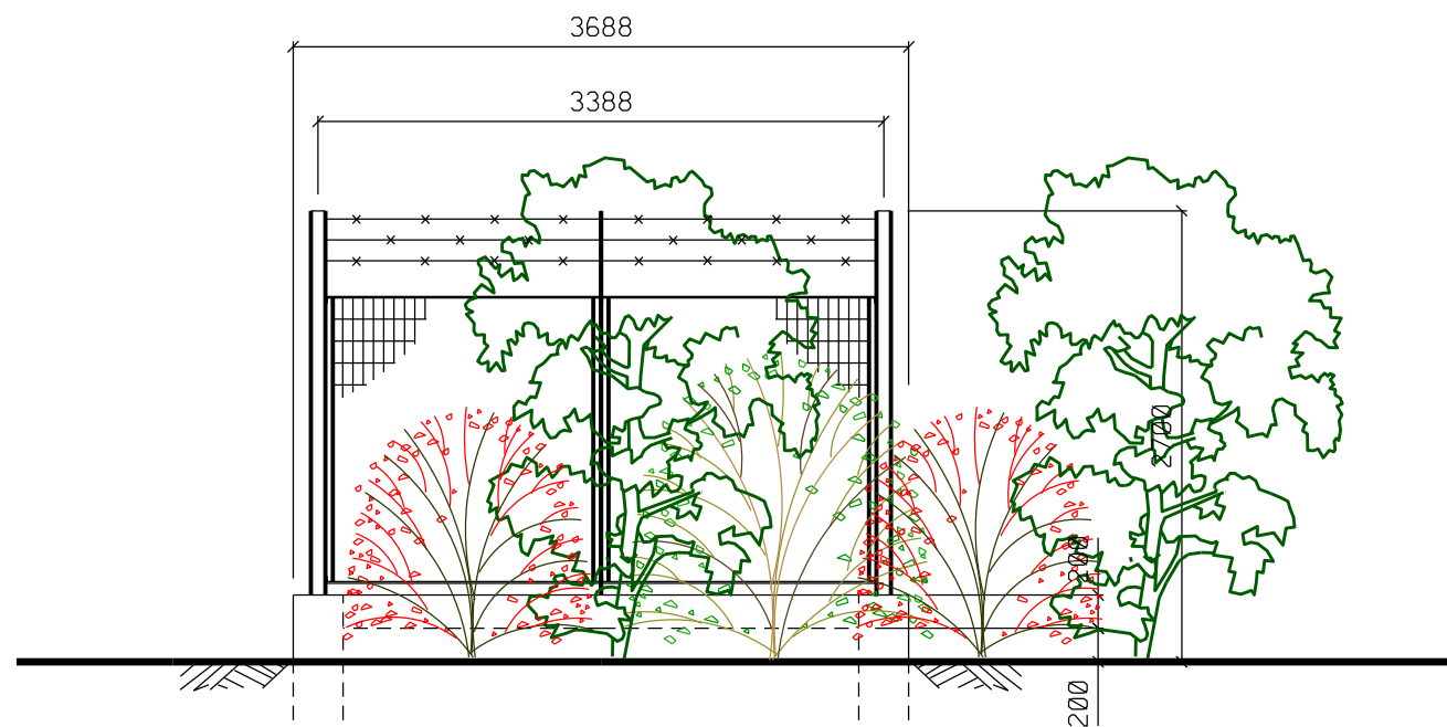
PROSPETTO C
