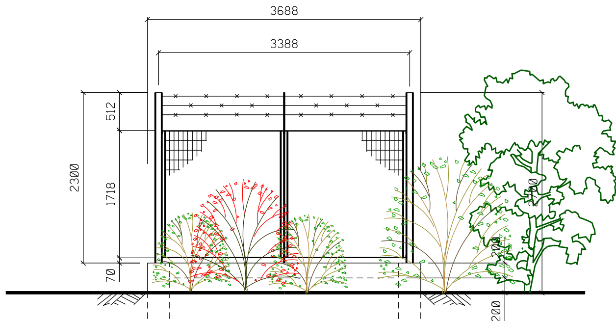
PROSPETTO B
