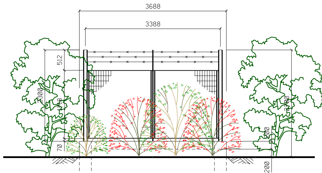
PROSPETTO C
