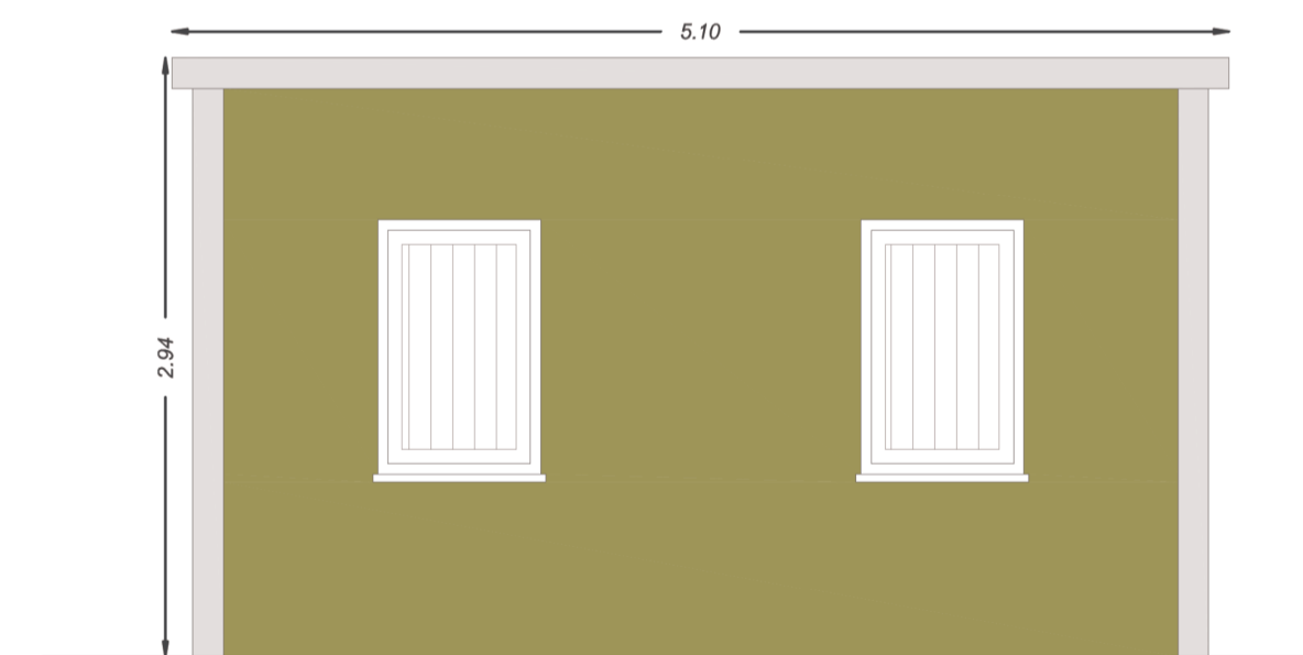
Prospetto DX
