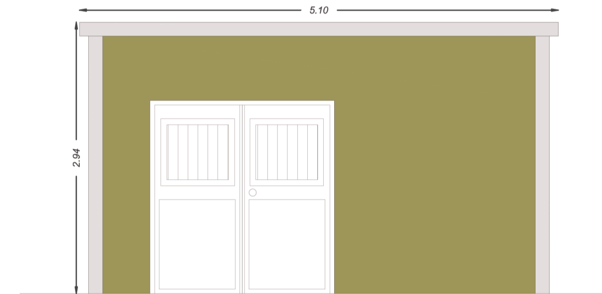
Prospetto anteriore
