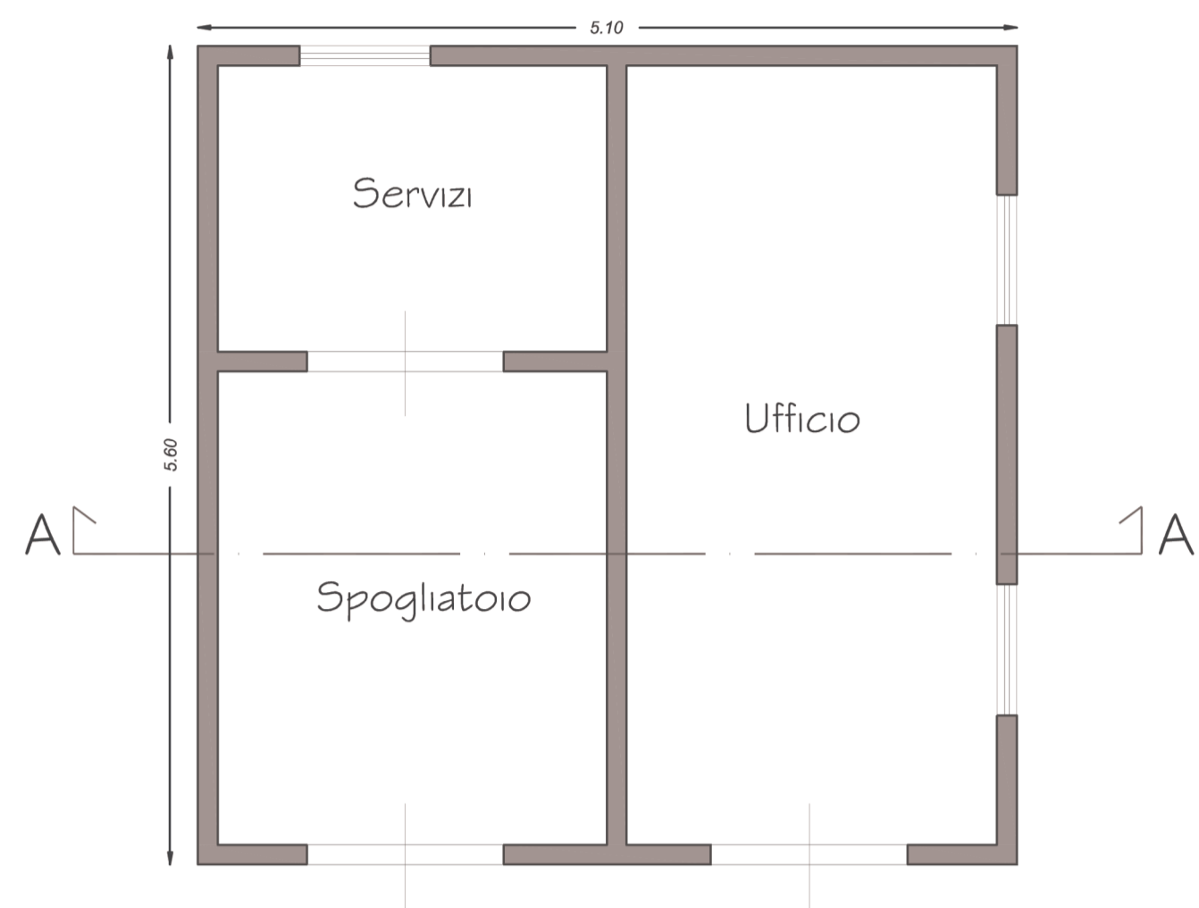
Pianta locale Ufficio e Servizi
