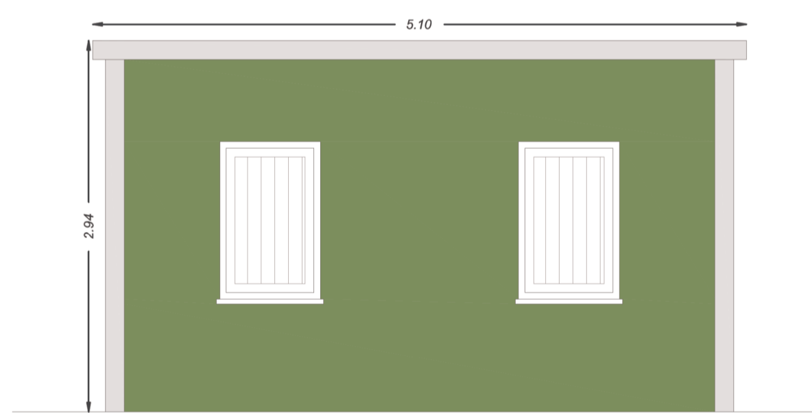
Prospetto DX
