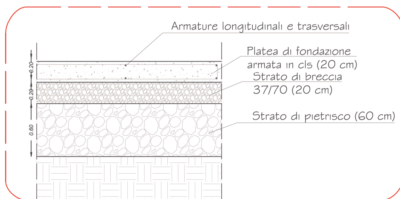
Dettaglio fondazione
