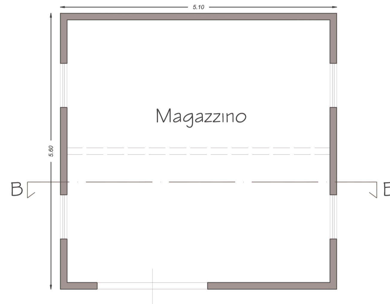
Pianta locale Magazzino
