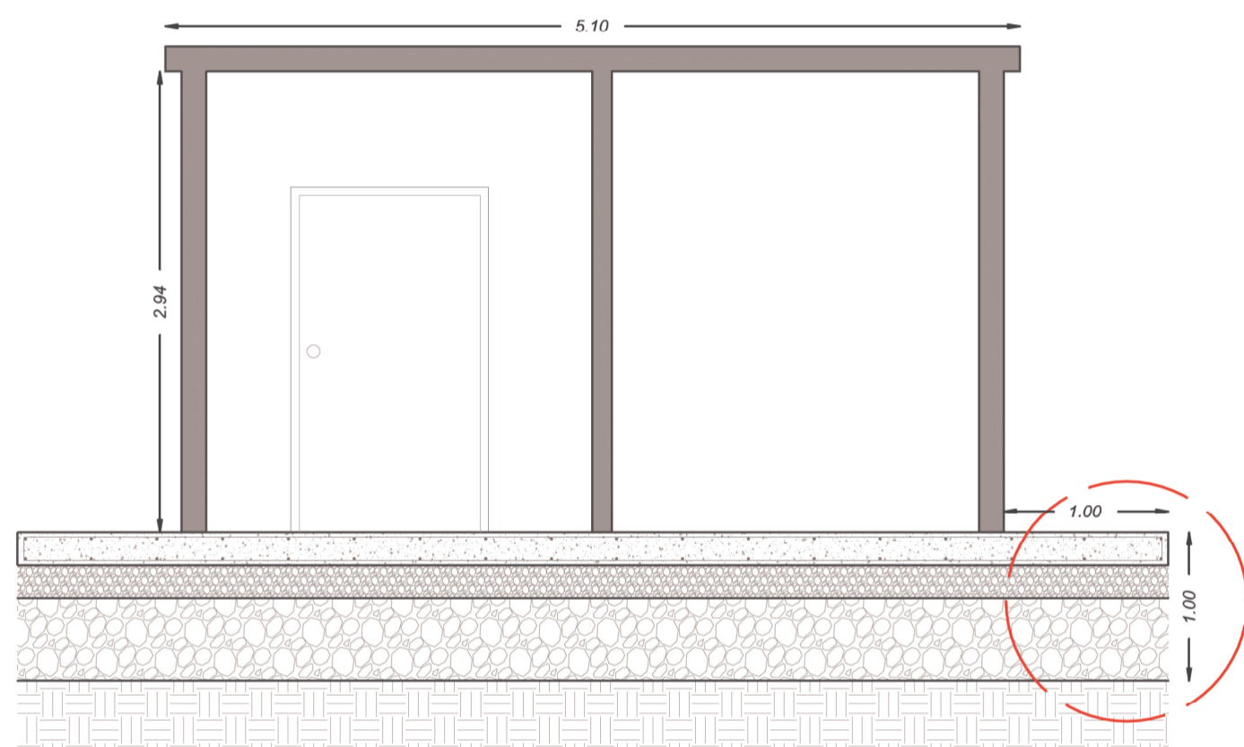
Sezione A-A
