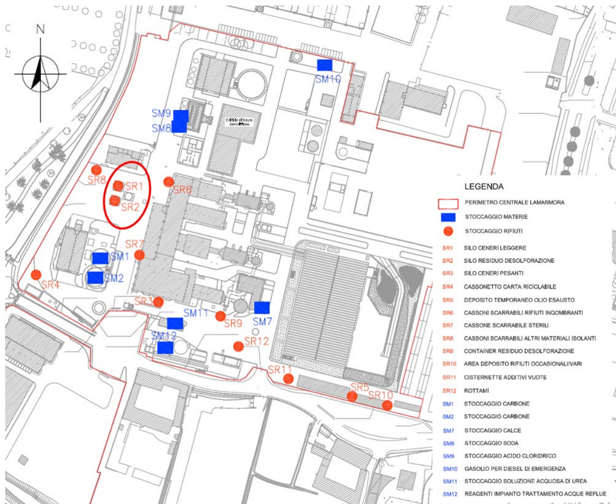
Figura 6.1: Stralcio della Planimetria con Individuazione delle Aree per lo Stoccaggio di Materie Prime e Rifiuti (Allegato B.22 alla Documentazione di Riesame AIA, 2019)
