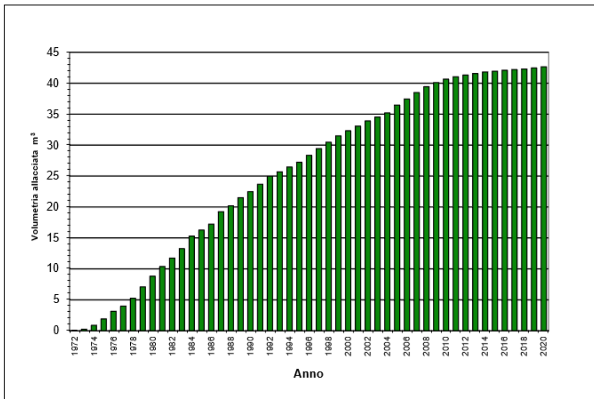
Figura 2.3: Volumetria Allacciata alla Rete di Teleriscaldamento, Anni 1972-2020
