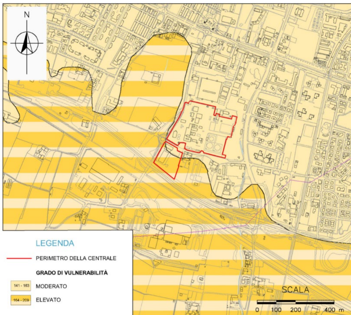
Figura 4.4: Vulnerabilità delle Acque Sotterranee (Comune di Brescia, 2018b)
