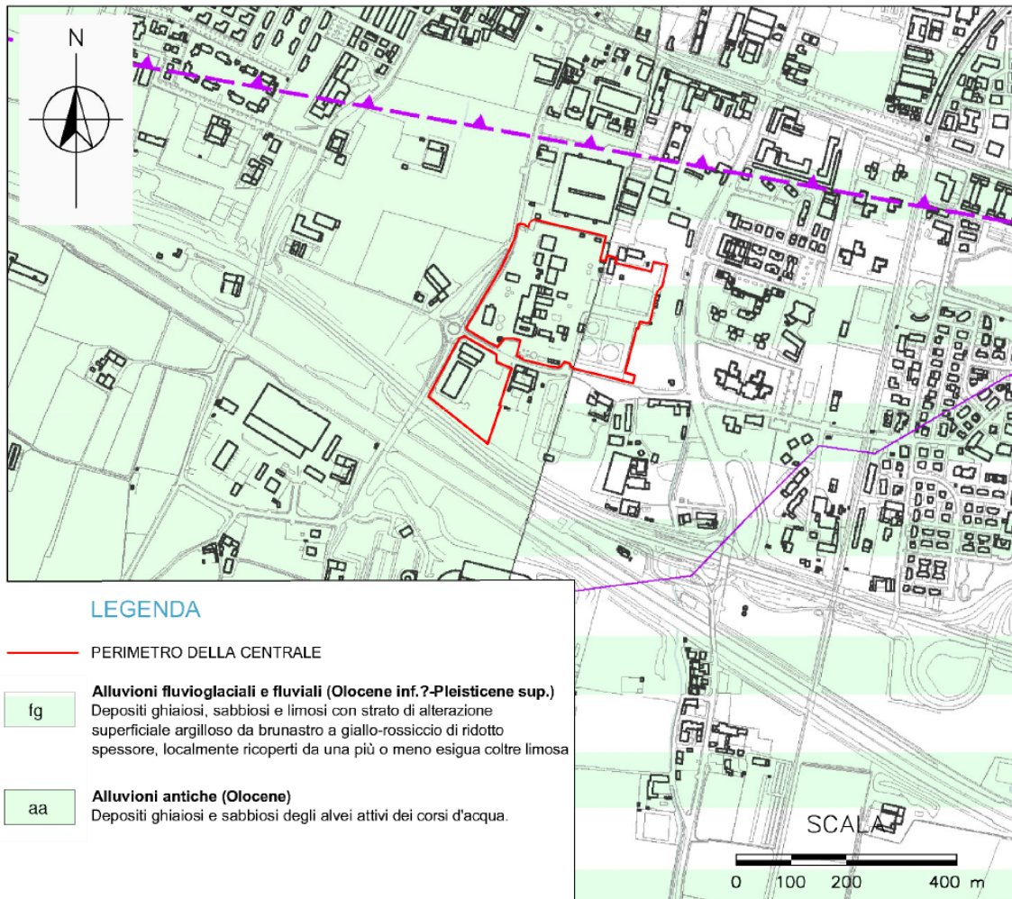
Figura 4.1: Geologia dell'Area di Interesse (Comune di Brescia, 2020a)
