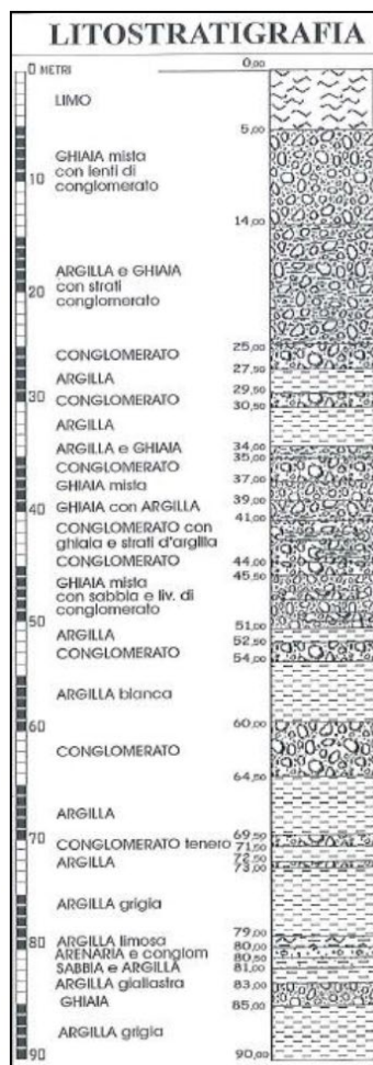
Figura 4.2: Litostratigrafia Pozzo Lamarmora A (ASM Brescia S.p.A. 2007)
