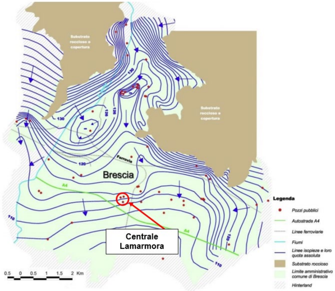
Figura 4.3: Direzione della Falda nel Territorio Comunale di Brescia (Comune di Brescia, 2020b)
