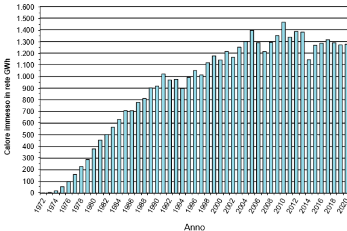
Figura 2.4: Crescita della Domanda di Calore per la Rete di Teleriscaldamento di Brescia
