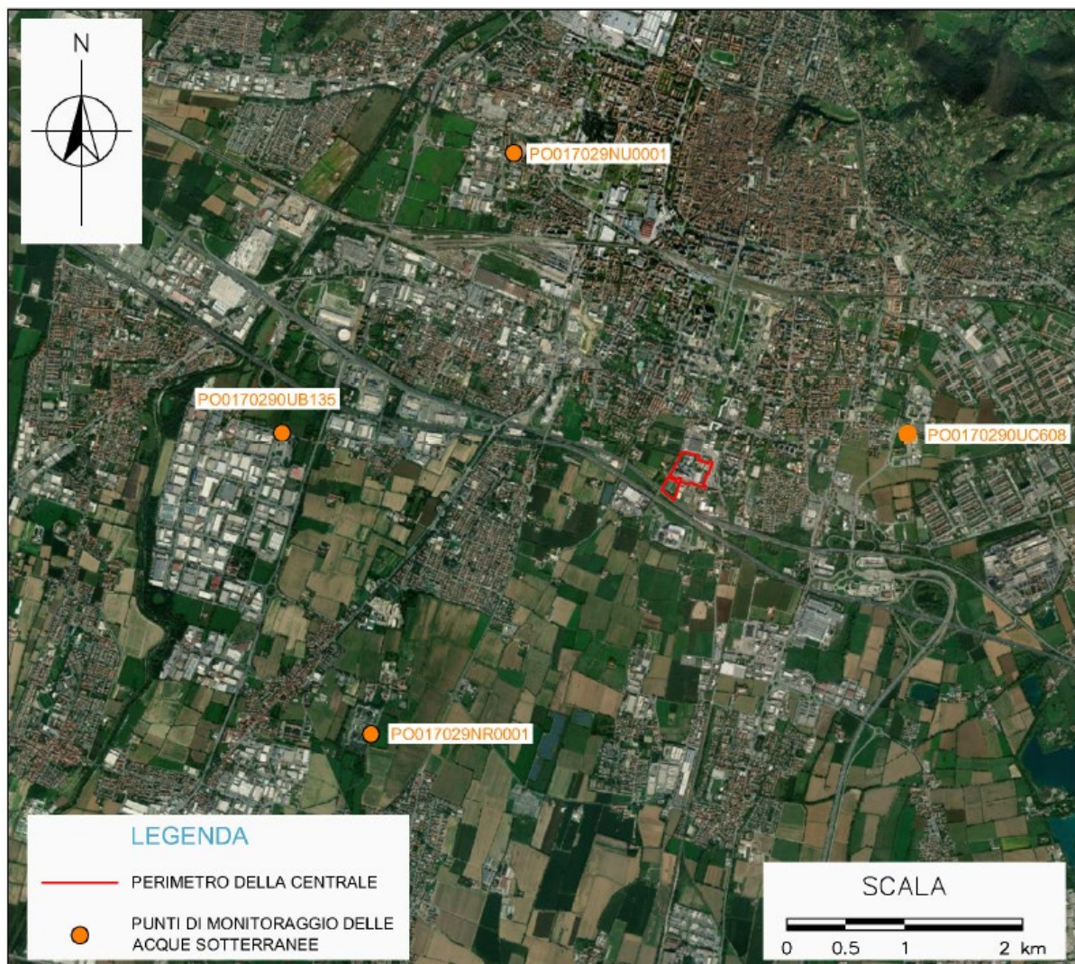
Figura 5.1: Pozzi Rete di Monitoraggio ARPA Lombardia
