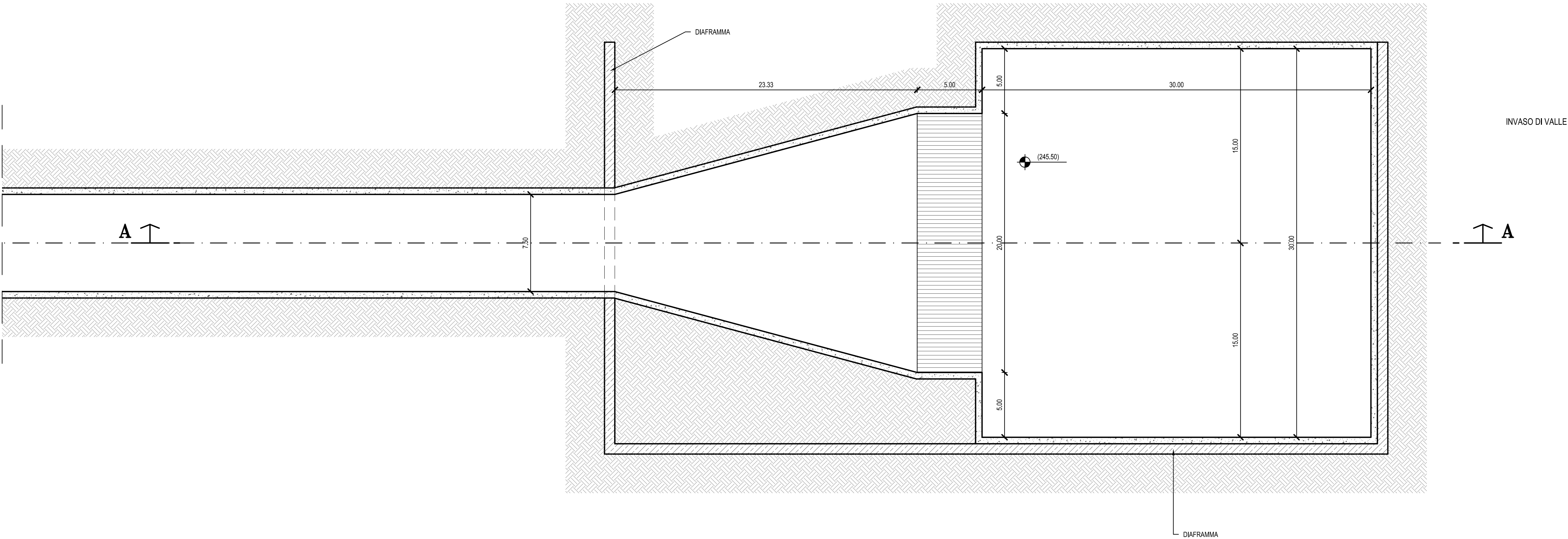
PIANTA 1:200
